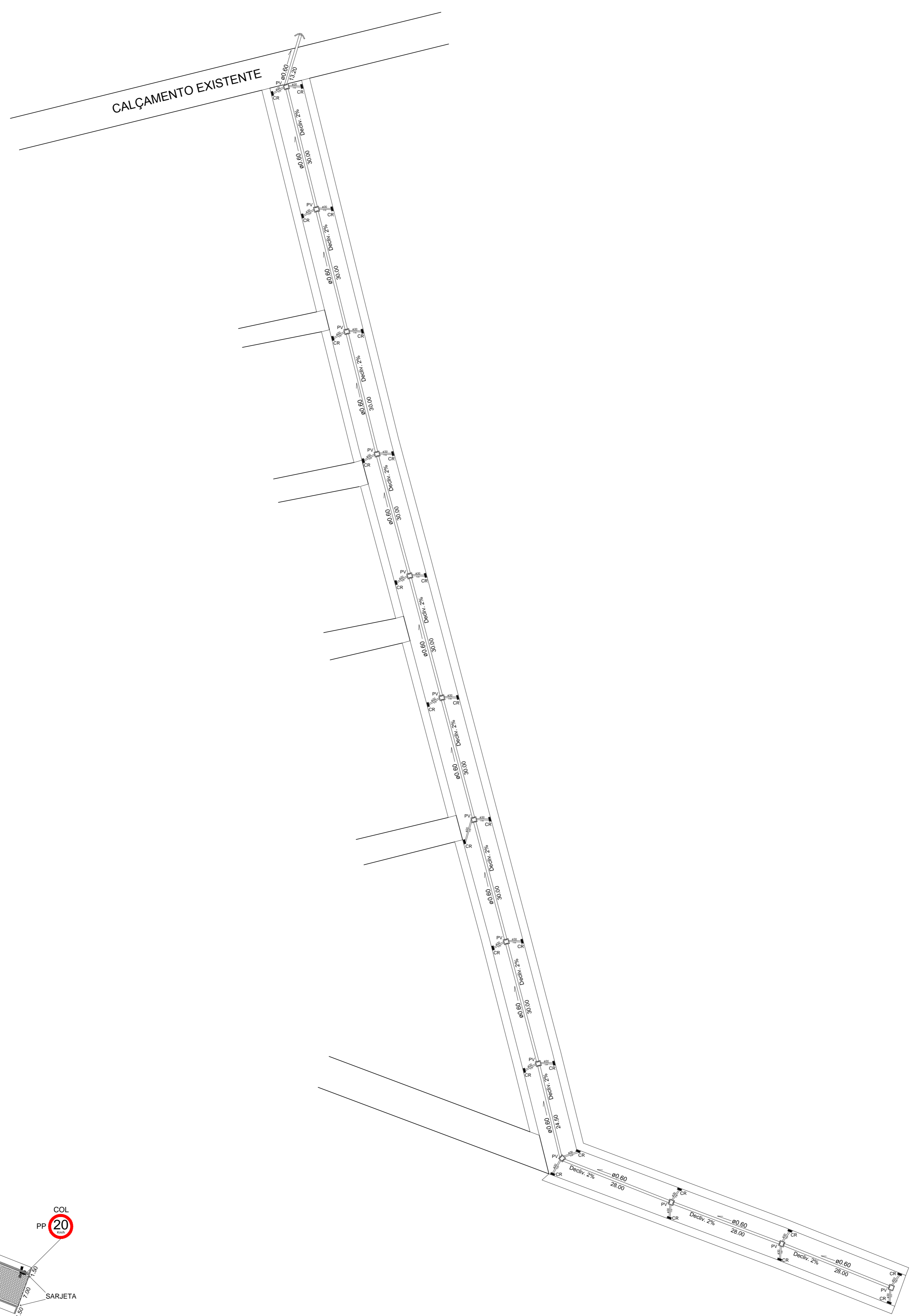
PLANTA BAIXA- DRENAGEM PLUVIAL ESCALA 1/750
