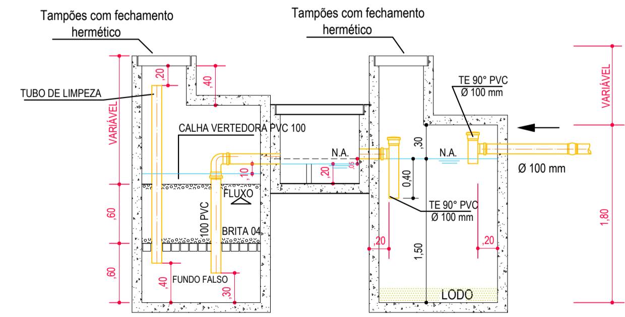
CORTE AA' Cotas em metros ESC. 1/50
