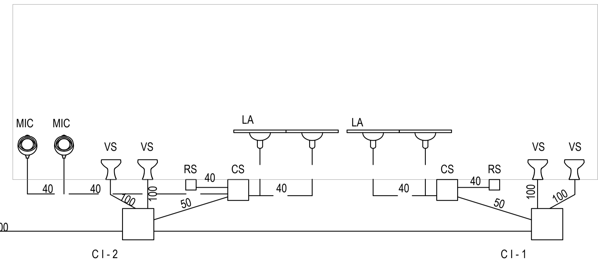
ESQUEMA VERTICAL
