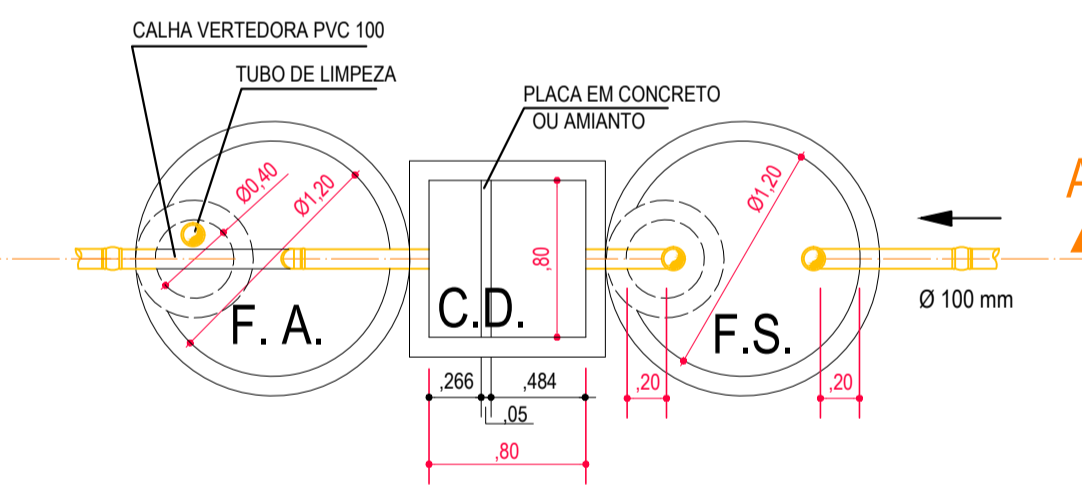
PLANTA BAIXA FOSSA SÉPTICA FILTRO ANAERÓBIO Cotas em metros ESC. 1/50
