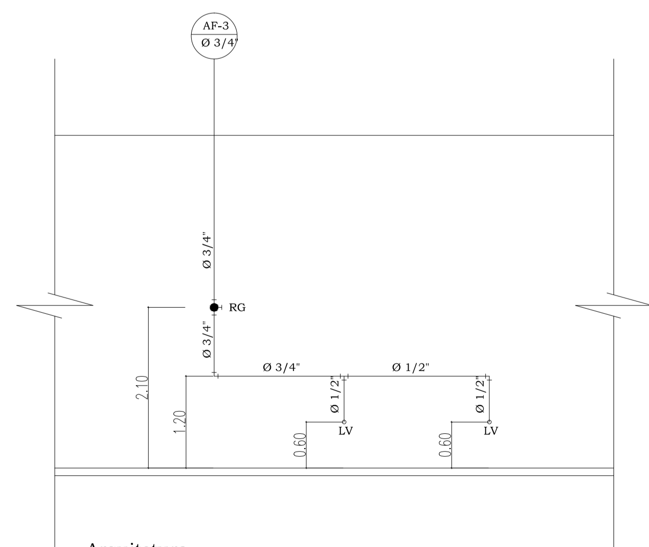
Arquitetura ESQUEMA VERTICAL - 03 (AF-3) Cotas em metro. Escala 1/50
