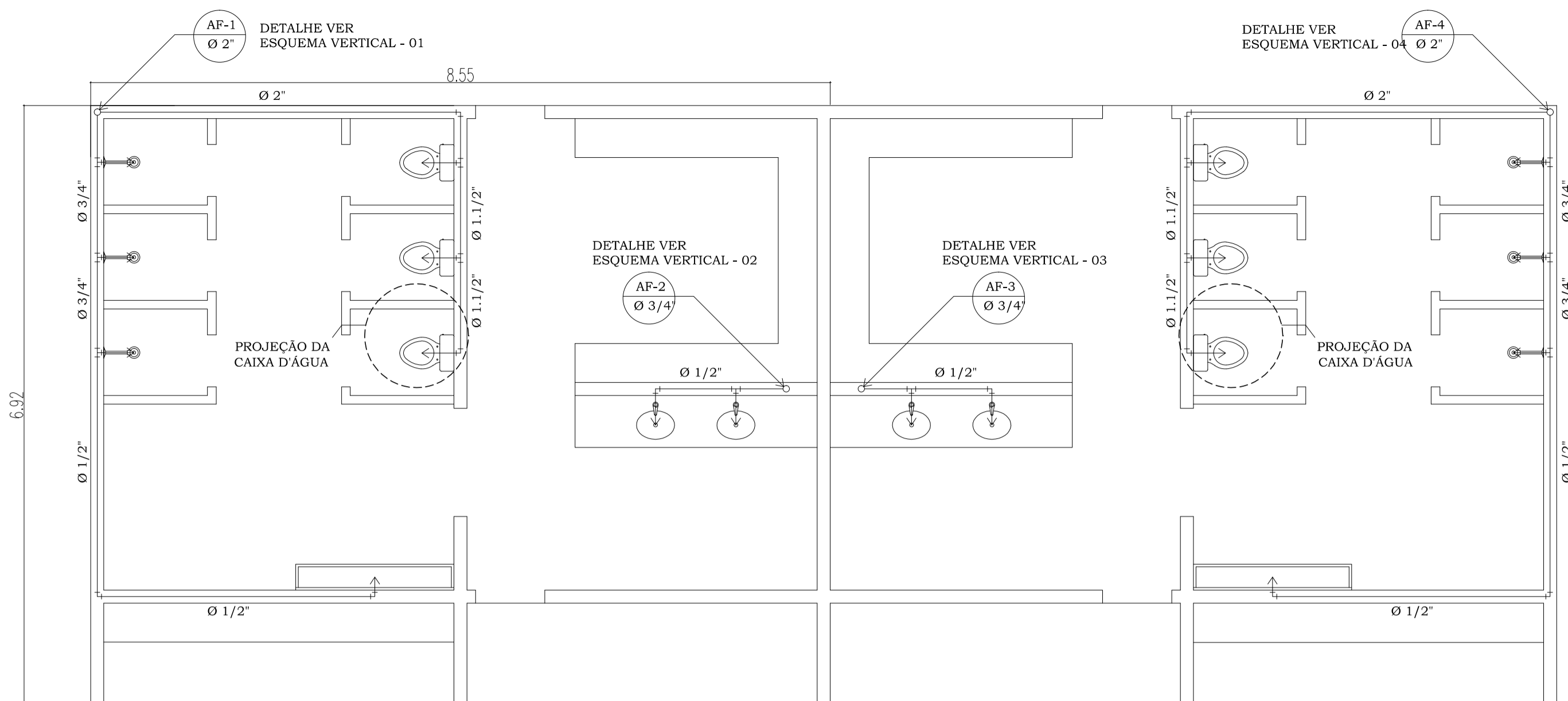
Arquitetura PLANTA BAIXA - INST. HIDRÁULICA Cotas em metro. Escala 1/50
