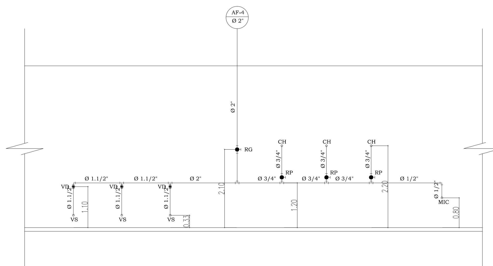
Arquitetura ESQUEMA VERTICAL - 04 (AF-4) Cotas em metro. Escala 1/50
