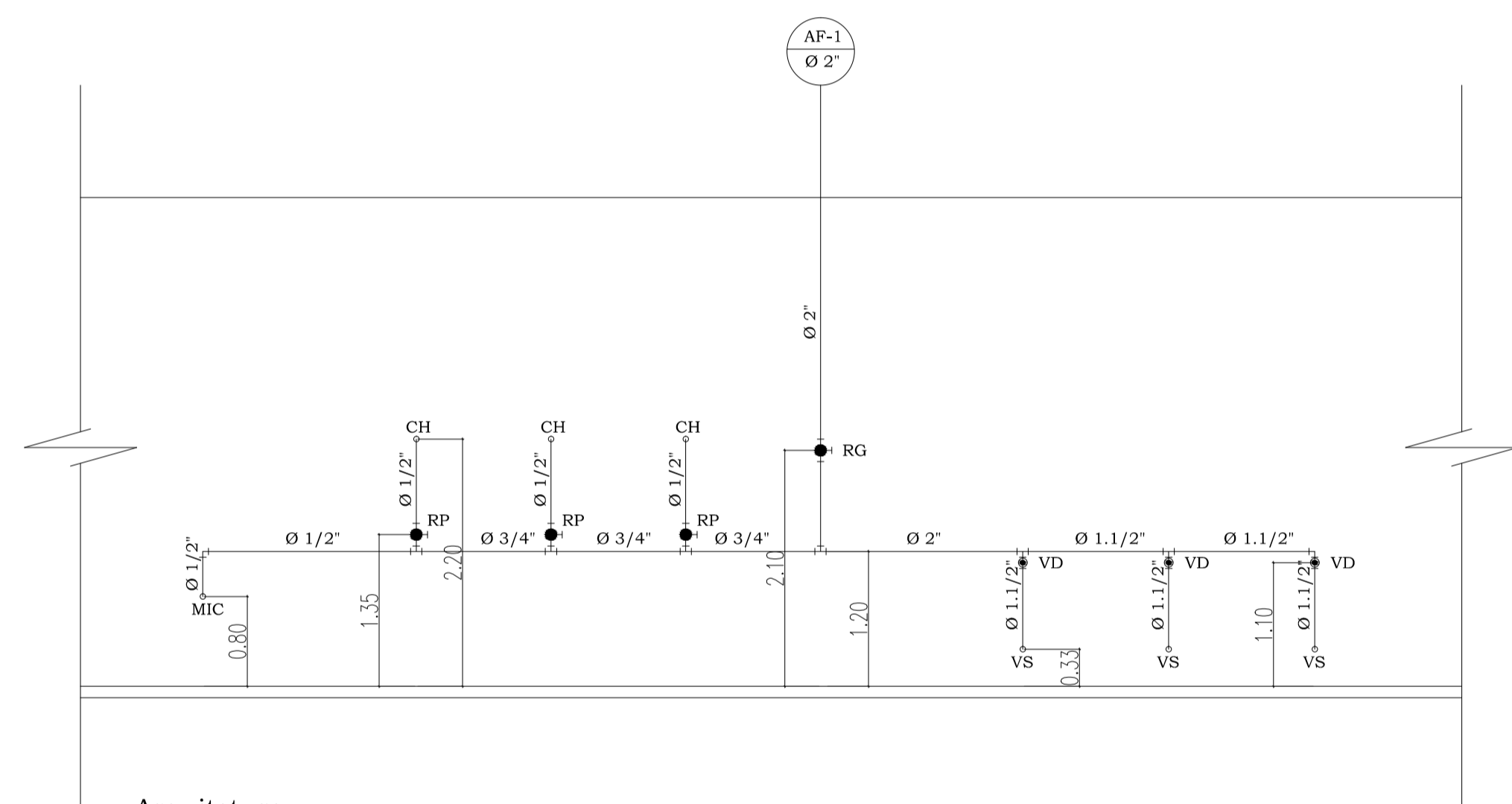
Arquitetura ESQUEMA VERTICAL - 01 (AF-1) Cotas em metro. Escala 1/50
