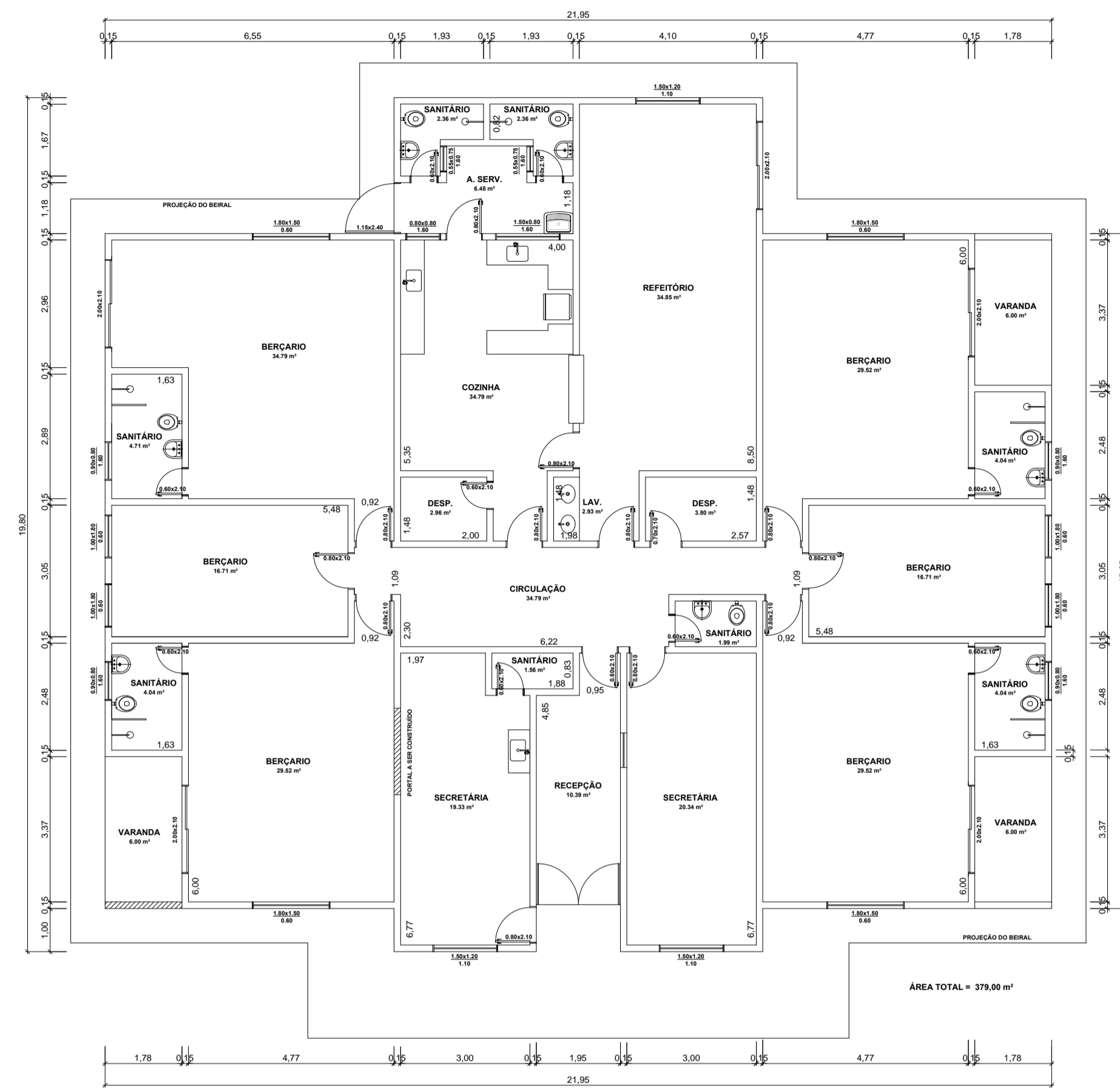
PLANTA BAIXA ESC.: 1/100
