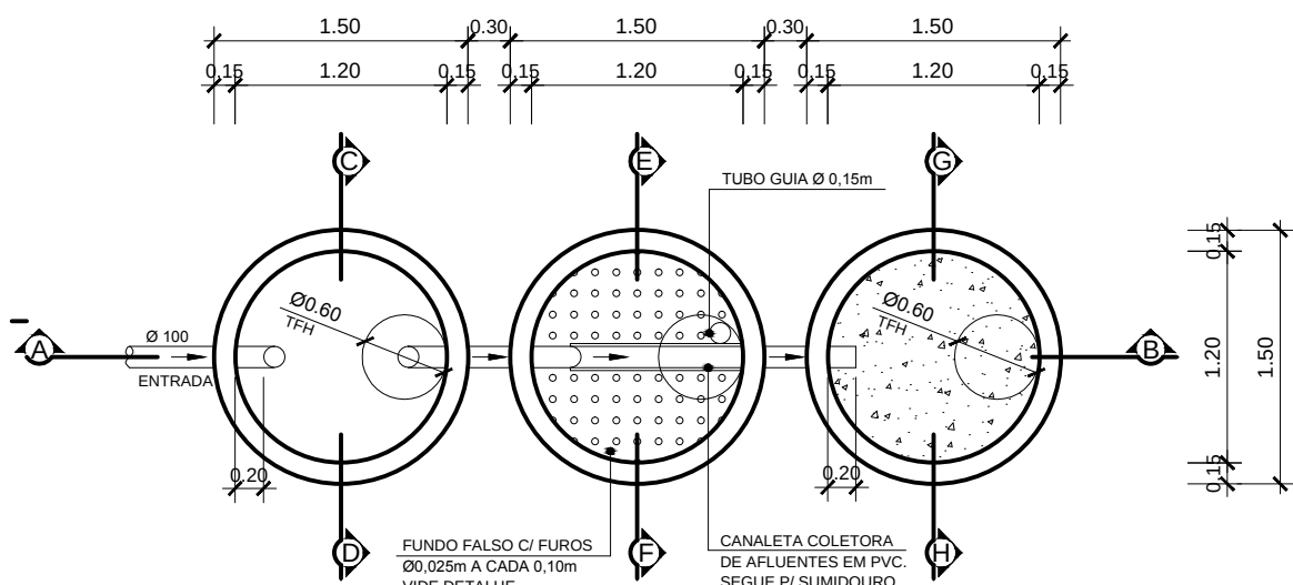
Arquitetura DETALHE 02 - Fossa, Filtro e Sumidouro Cotas em metro. Escala 1/50
