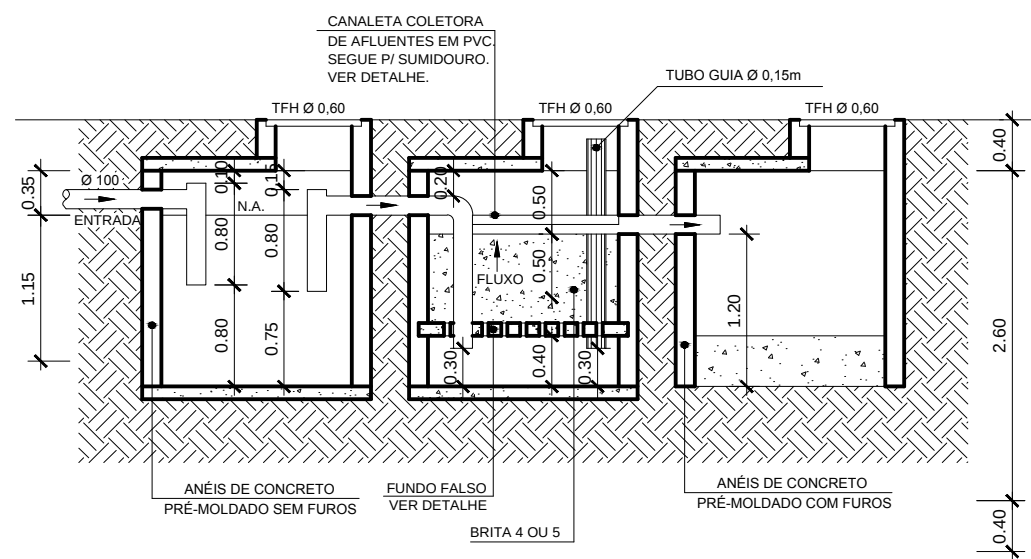
Arquitetura CORTE - AB - Fossa, Filtro e Sumidouro Cotas em metro. Escala 1/50
