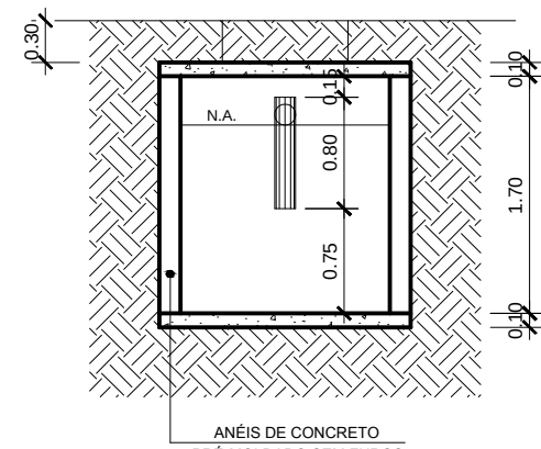
Arquitetura CORTE - CD - Fossa Cotas em metro. Escala 1/50
