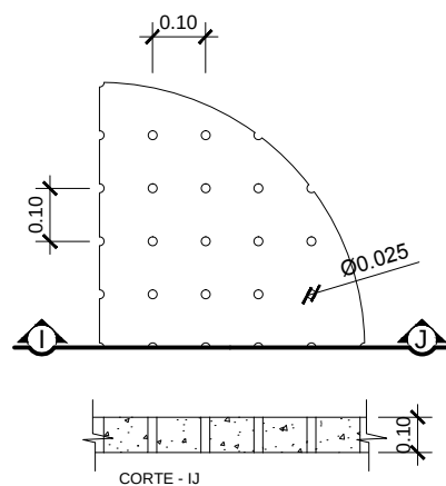
Arquitetura DETALHE - Fundo Falso Cotas em metro.
