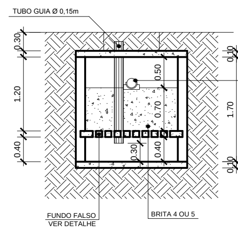
Arquitetura CORTE - EF - Filtro Cotas em metro. Escala 1/50
