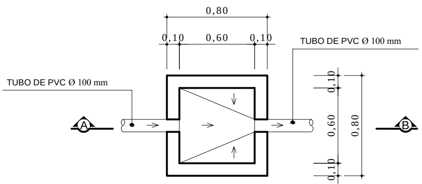
Arquitetura DETALHE 01 - Caixa de Inspeção Cotas em metro. Escala 1/25
