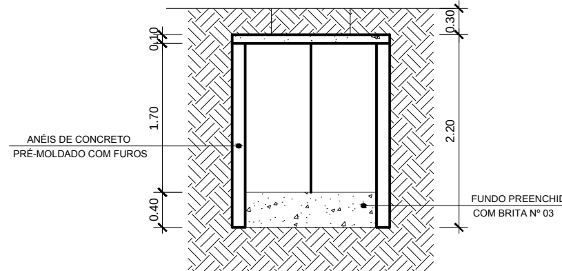
Arquitetura CORTE - GH - Sumidouro Cotas em metro. Escala 1/50
