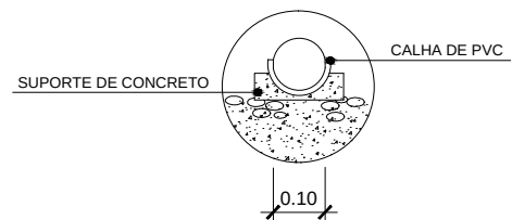
Arquitetura DETALHE - Canaleta Cotas em metro.
