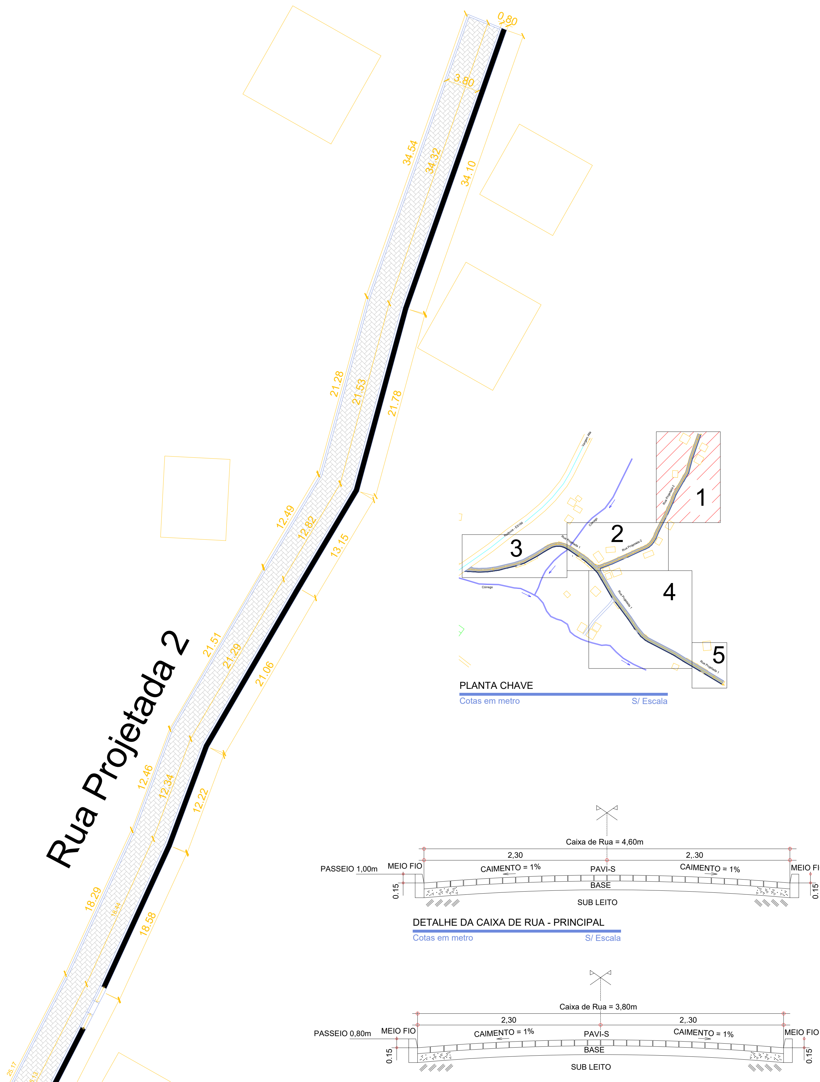
PLANTA BAIXA - PAVIMENTAÇÃO Cotas em metro Escala - 1/250
