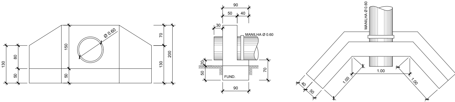
DETALHE BOCA - BSTC Cotas em metro Escala - 1/100
