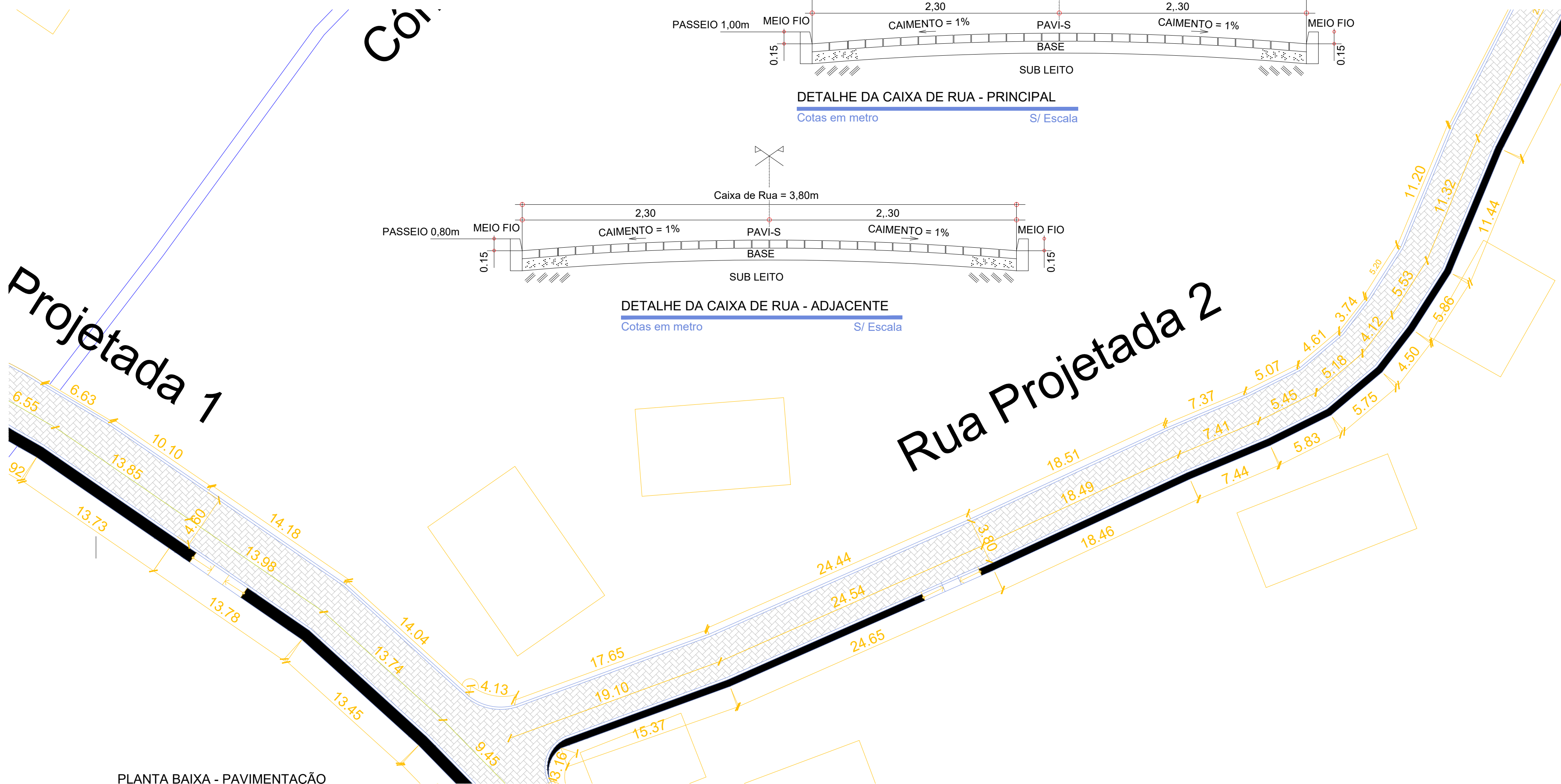
PLANTA BAIXA - PAVIMENTAÇÃO Cotas em metro Escala - 1/250
