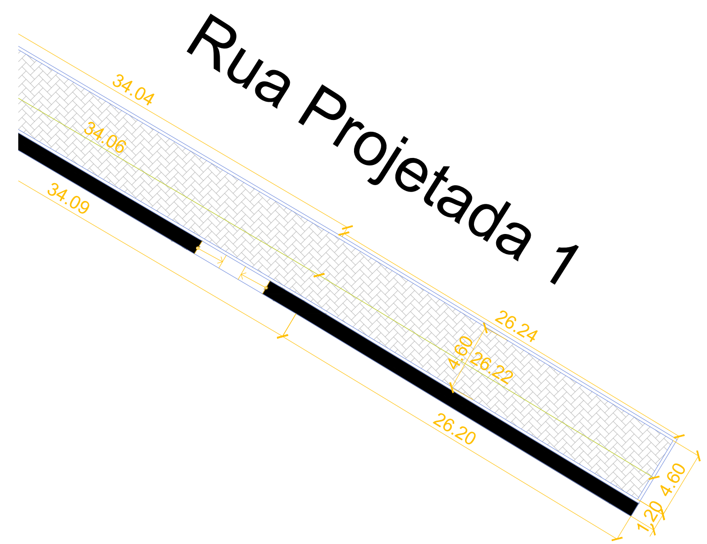
PLANTA BAIXA - PAVIMENTAÇÃO Cotas em metro Escala - 1/250
