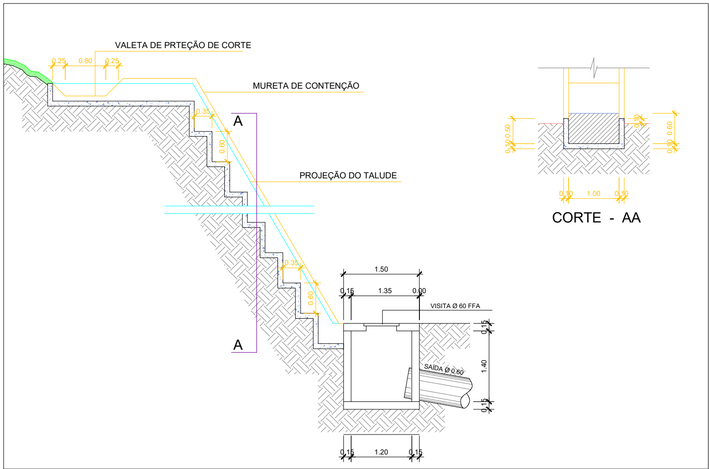
DETALHE - DESCIDA D'ÁGUA EM DEGRAUS E VALETA DE PROTEÇÃO DE CORTE Cotas em metro Escala - 1/75
