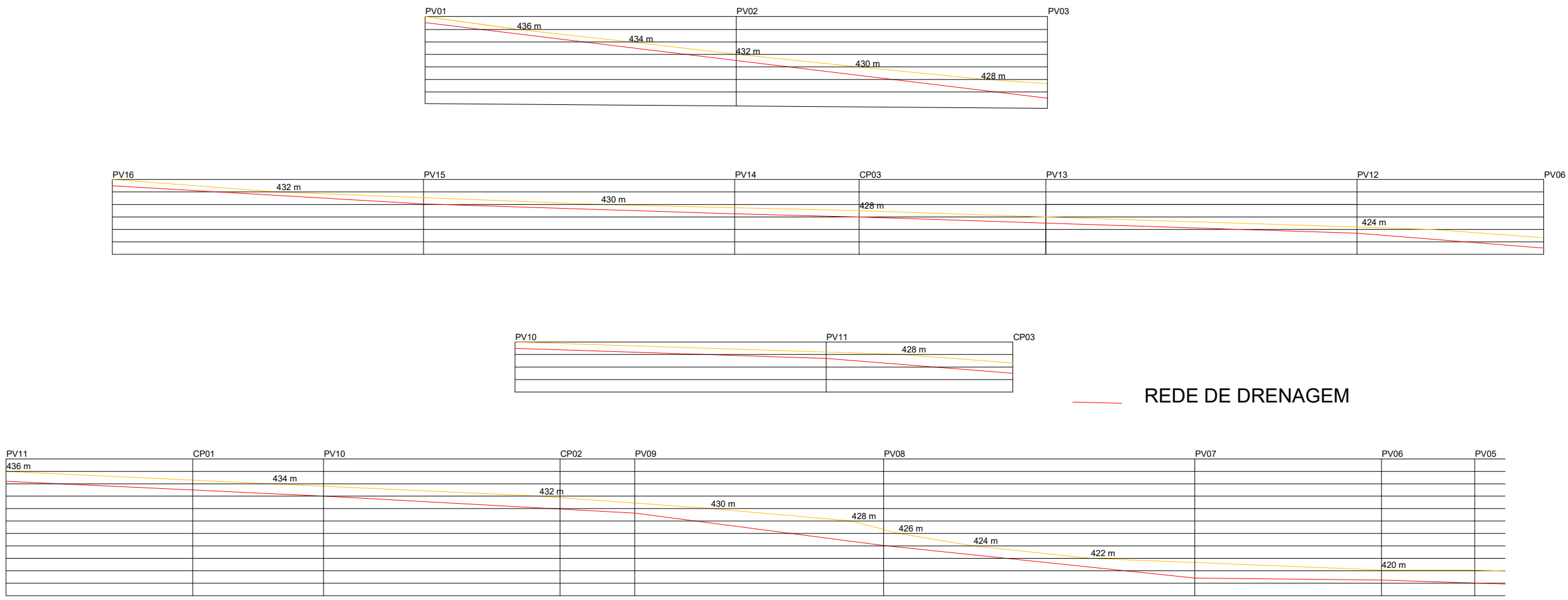
PERFIL DE ELEVÇÃO - DETALHE DA DRENAGEM E ESGOTO Cotas em metro Escala - 1/700
