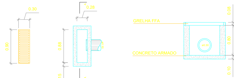
DETALHE CAIXA-RAIO Cotas em metro Escala - 1/50
