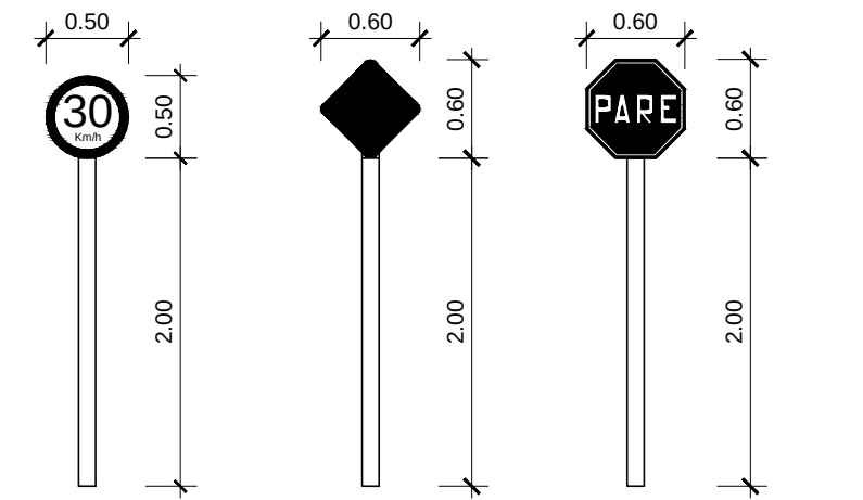
DETALHE - PLACAS Cotas em metro. Escala - 1/50
