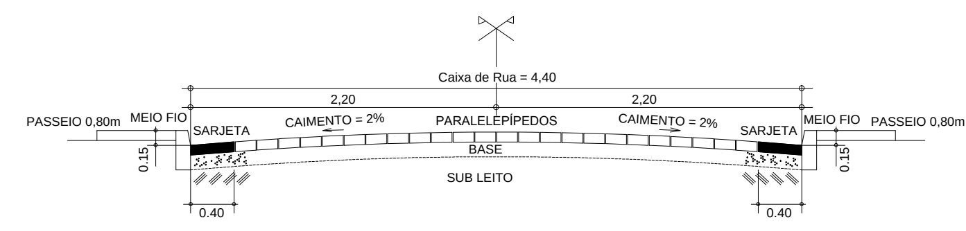
SEÇÃO TRANSVERSAL Cotas em metro. Escala - 1/50
