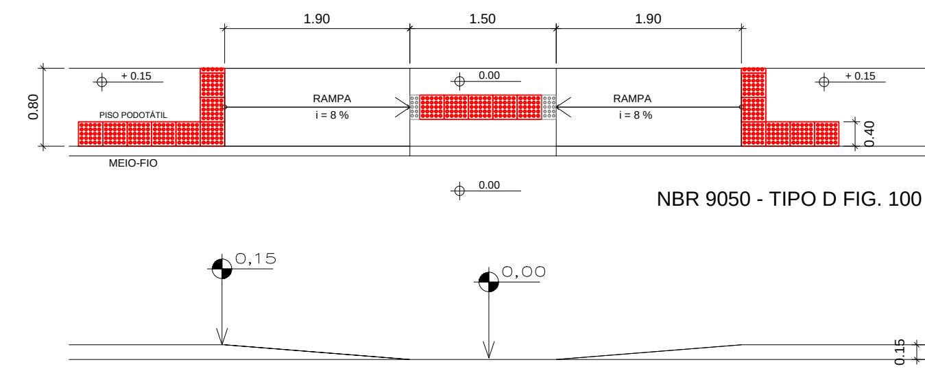
DET - PASSEIO - RAMPA DE ACESSIBILIDADE Cotas em metro. Escala - 1/50
