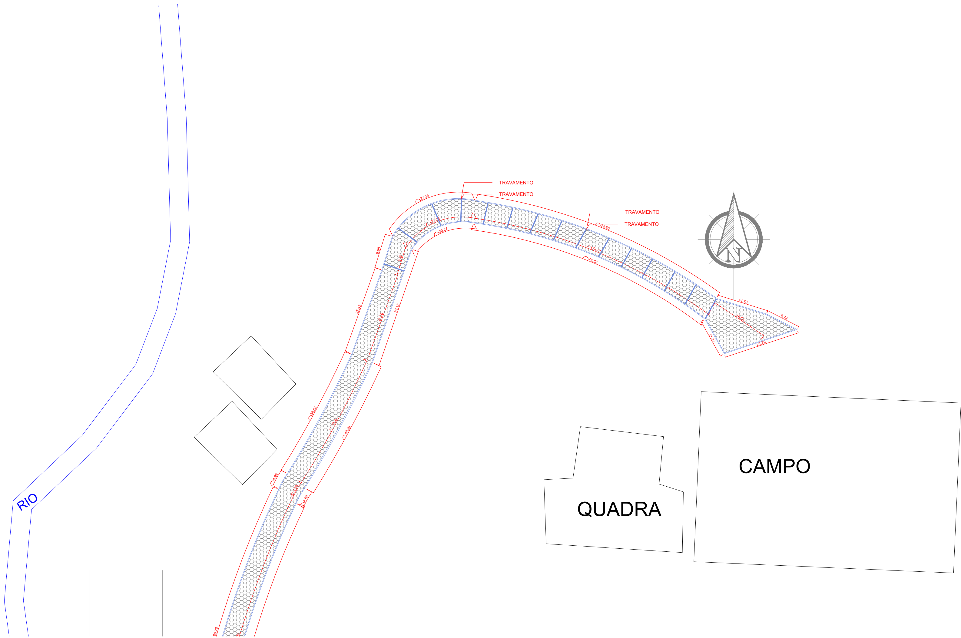
PLANTA BAIXA - PAVIMENTAÇÃO
