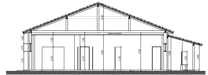
CORTE - BB ESC.: 1/75
