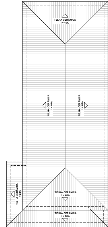
PLANTA DE COBERTURA ESC.: 1/125
