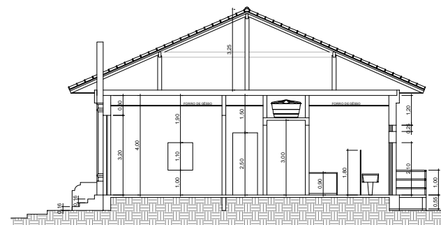
CORTE - BB ESC.: 1/75
