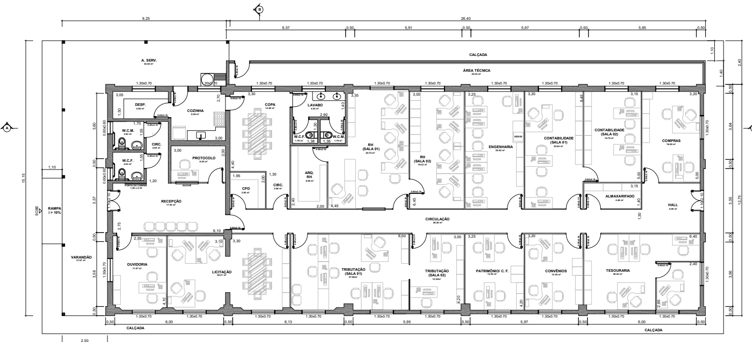
PLANTA BAIXA ESC.: 1/75
