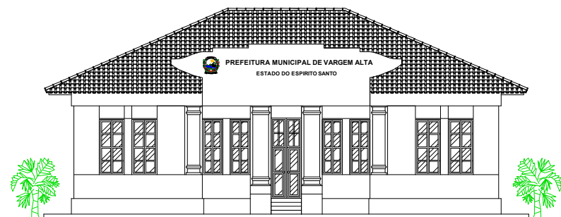
FACHADA ESC.: 1/75
