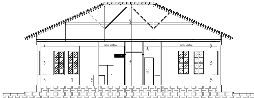
CORTE - AA ESC.: 1/75
