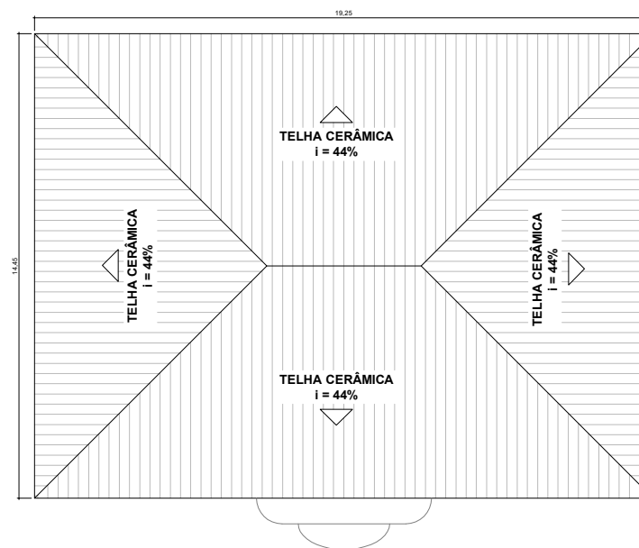
PLANTA DE COBERTURA ESC.: 1/75
