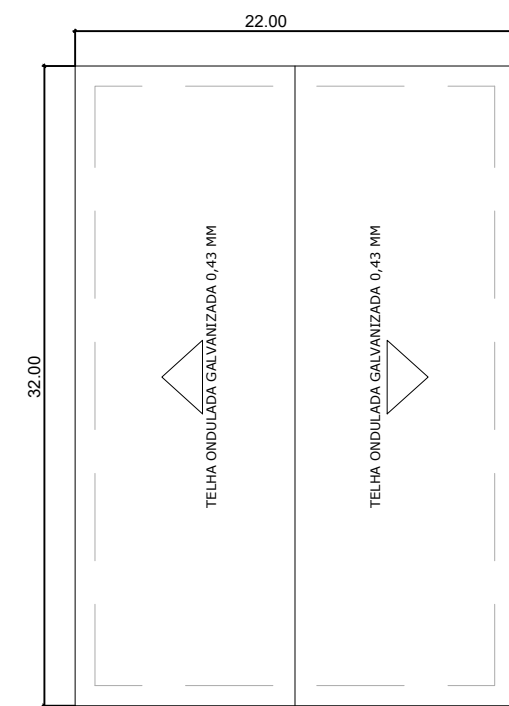
PLANTA TELHADO Cotas em metro. Escala - 1/350
