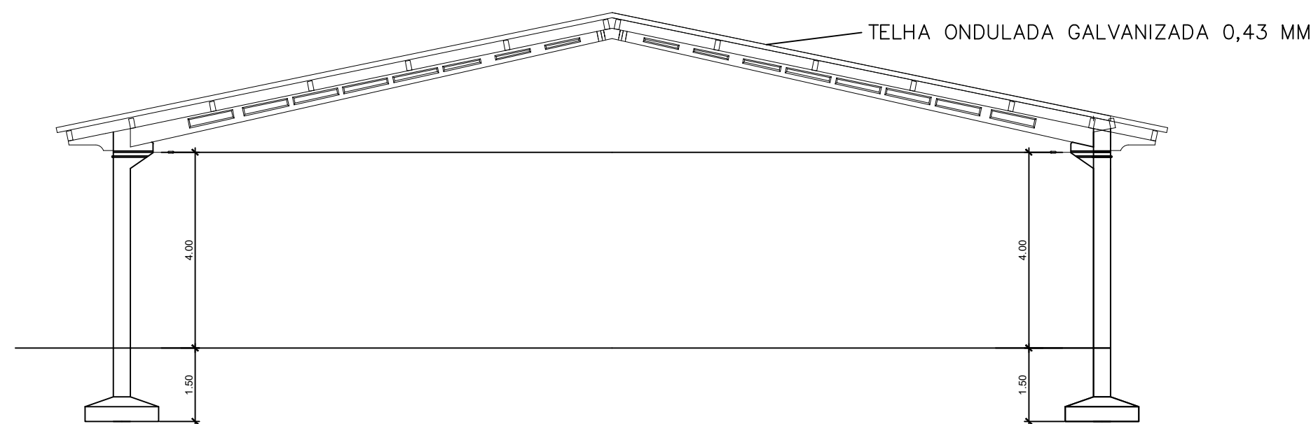
CORTE AA Cotas em metro. Escala - 1/100
