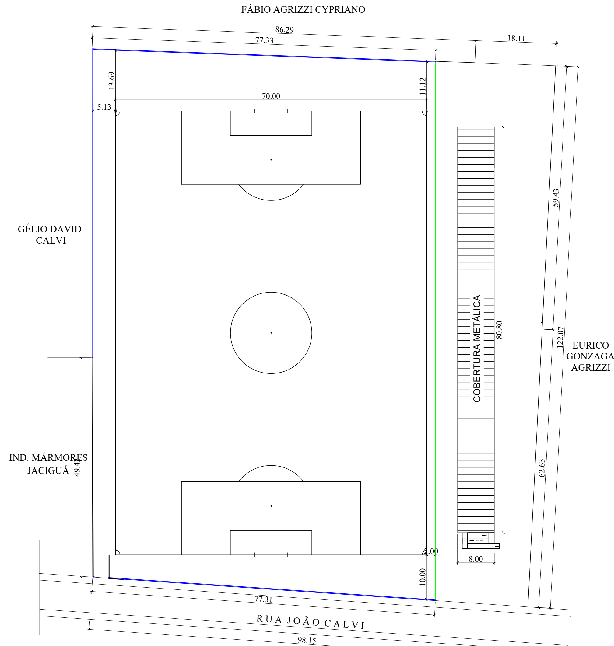
PLANTA DE SITUAÇÃO 1 : 500
