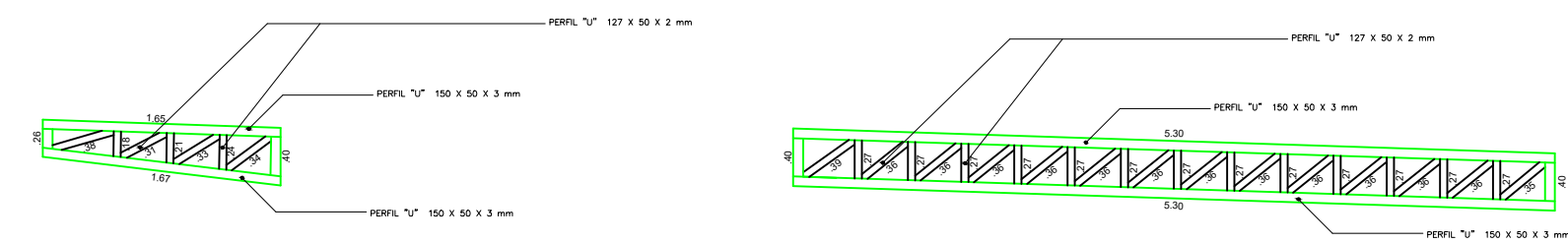
DETALHE TRELIÇA METÁLICA 1 : 50
