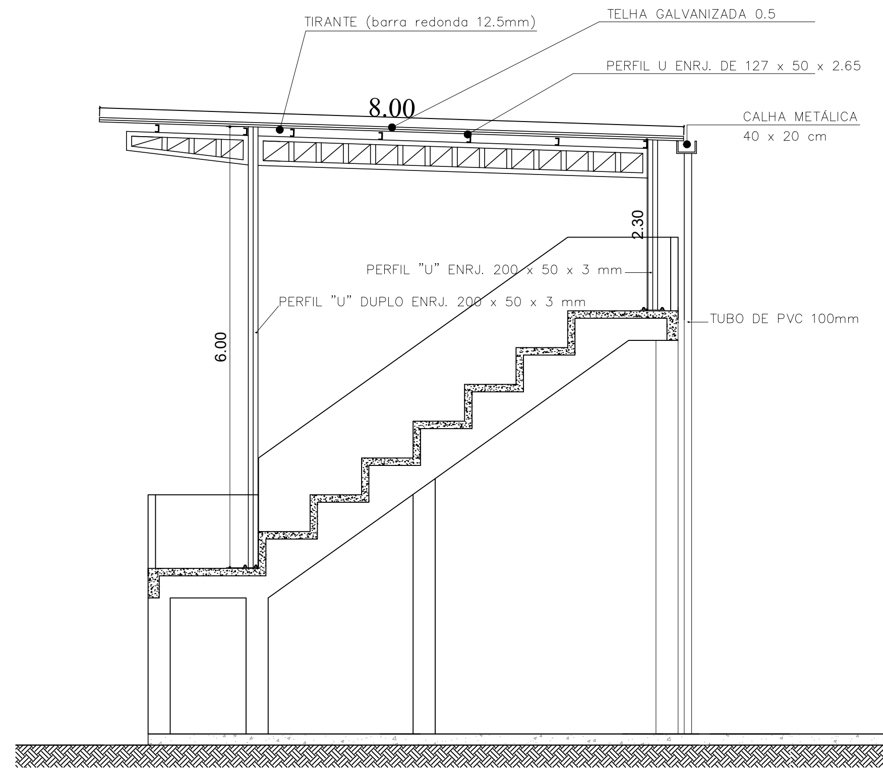
CORTE - A A 1 : 50
