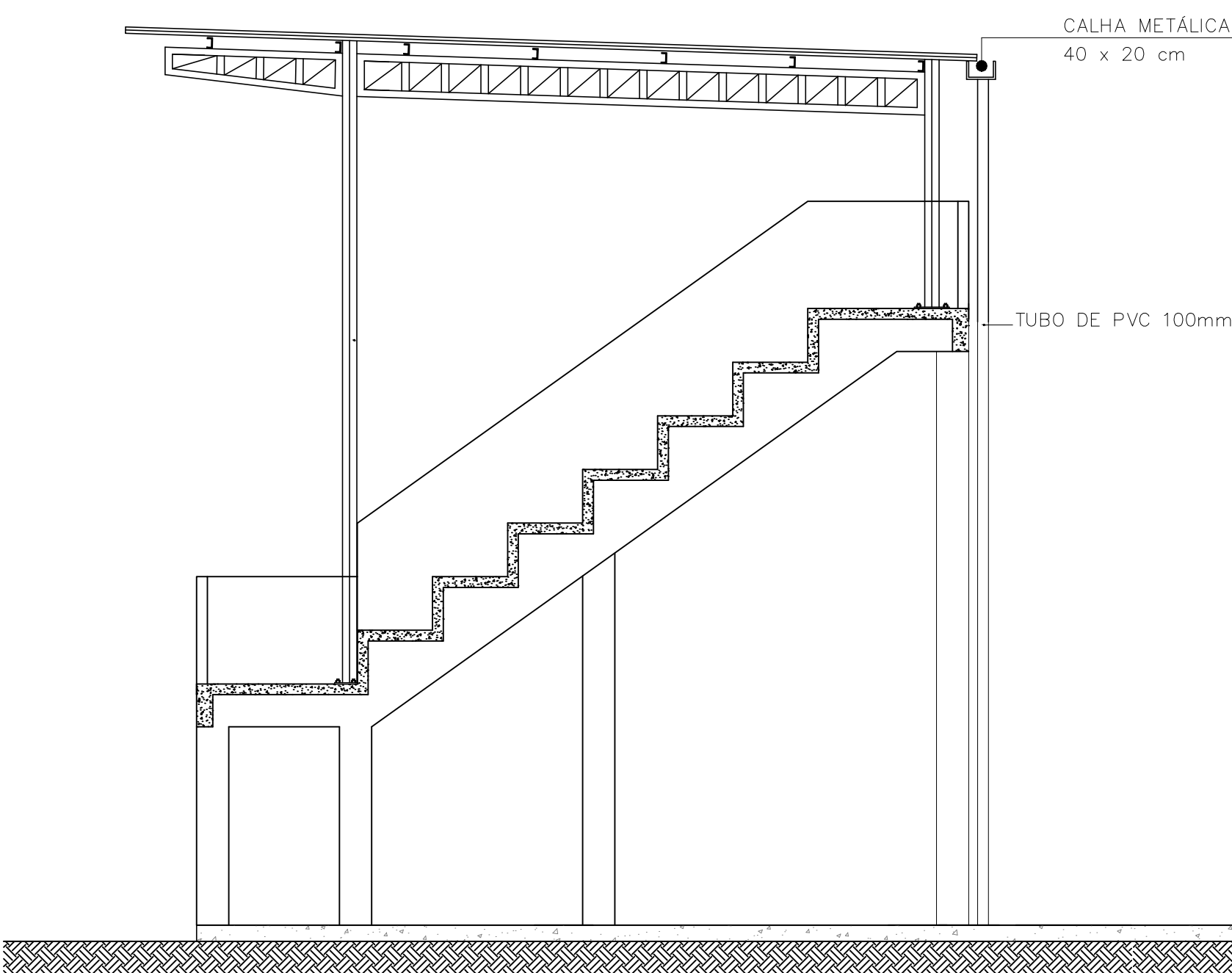
CORTE - A A TUBO DE DRENAGEM 1:50
