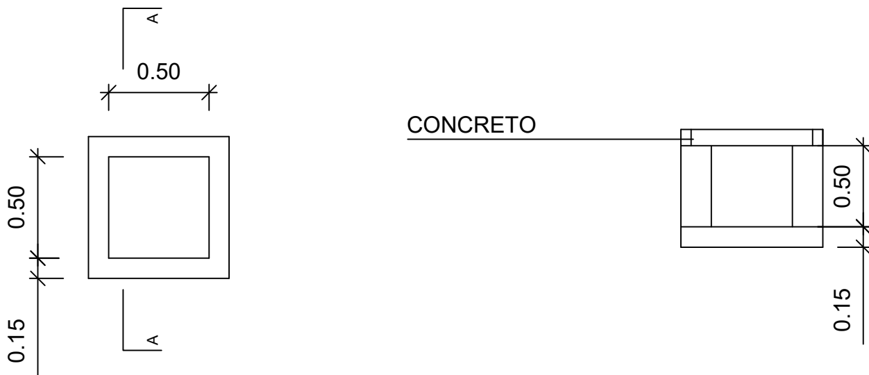
DET. CAIXA RALO ( D.1 0.50 x 0.50 x 0.50) ESC. 1/25
