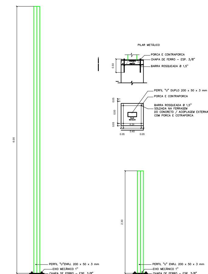
DETALHE DO PILAR METÁLICO 1 : 50
