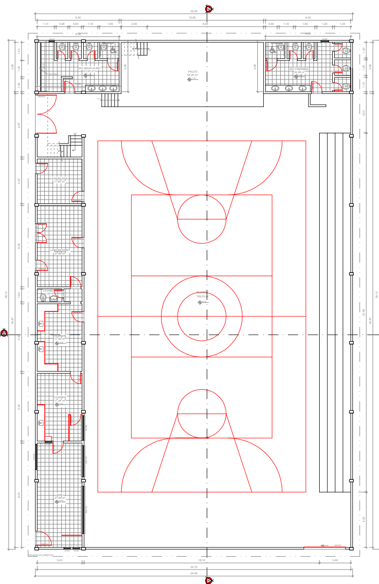
PLANTA BAIXA - PROPOSTA REFORMA 1/100
