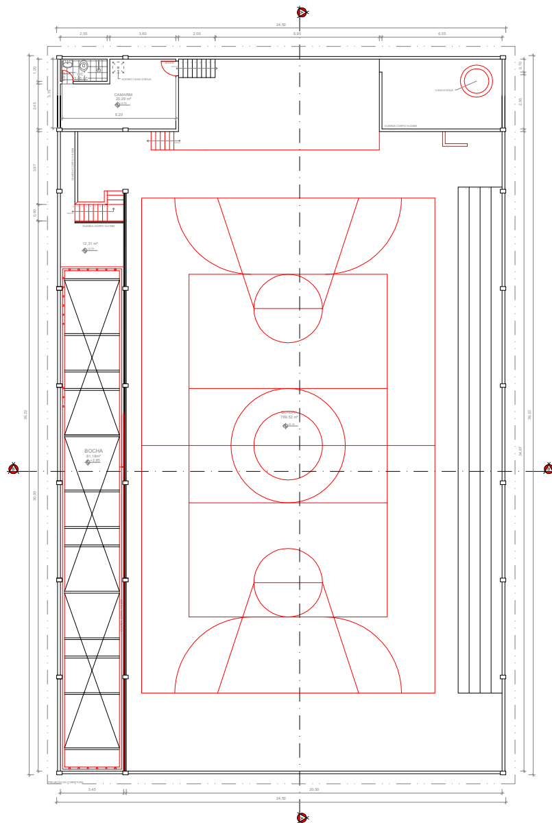
PLANTA BAIXA - 2º PAV. - PROPOSTA DE REFORMA 1/100
