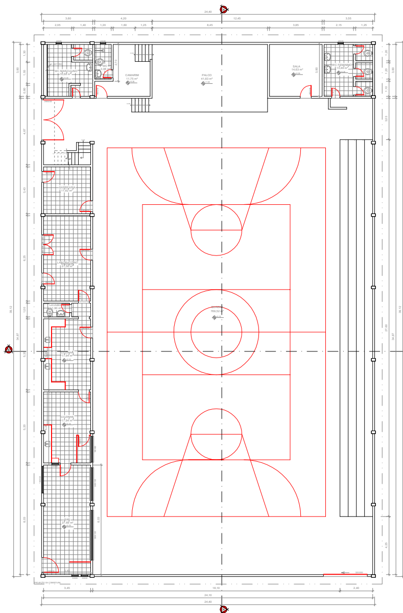
PLANTA BAIXA - PROJETO ATUAL 1/100
