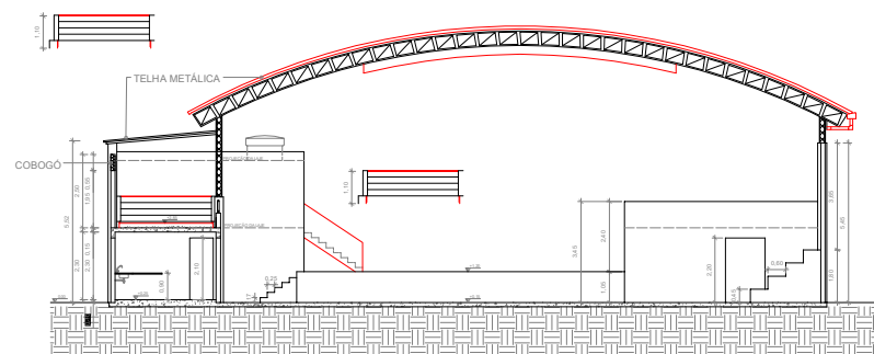
CORTE BB 1/100
