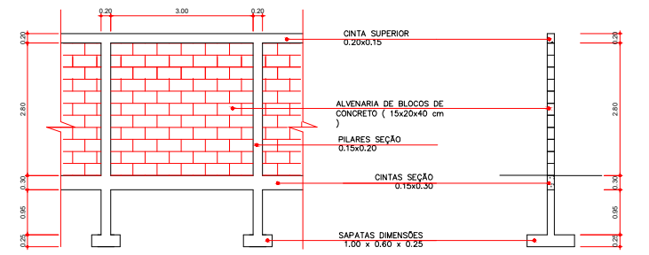
FACHADA ESCALA 1/50
