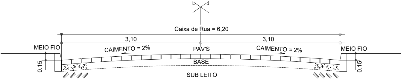
SEÇÃO TRANSVERSAL Cotas em metro. Escala - 1/50
