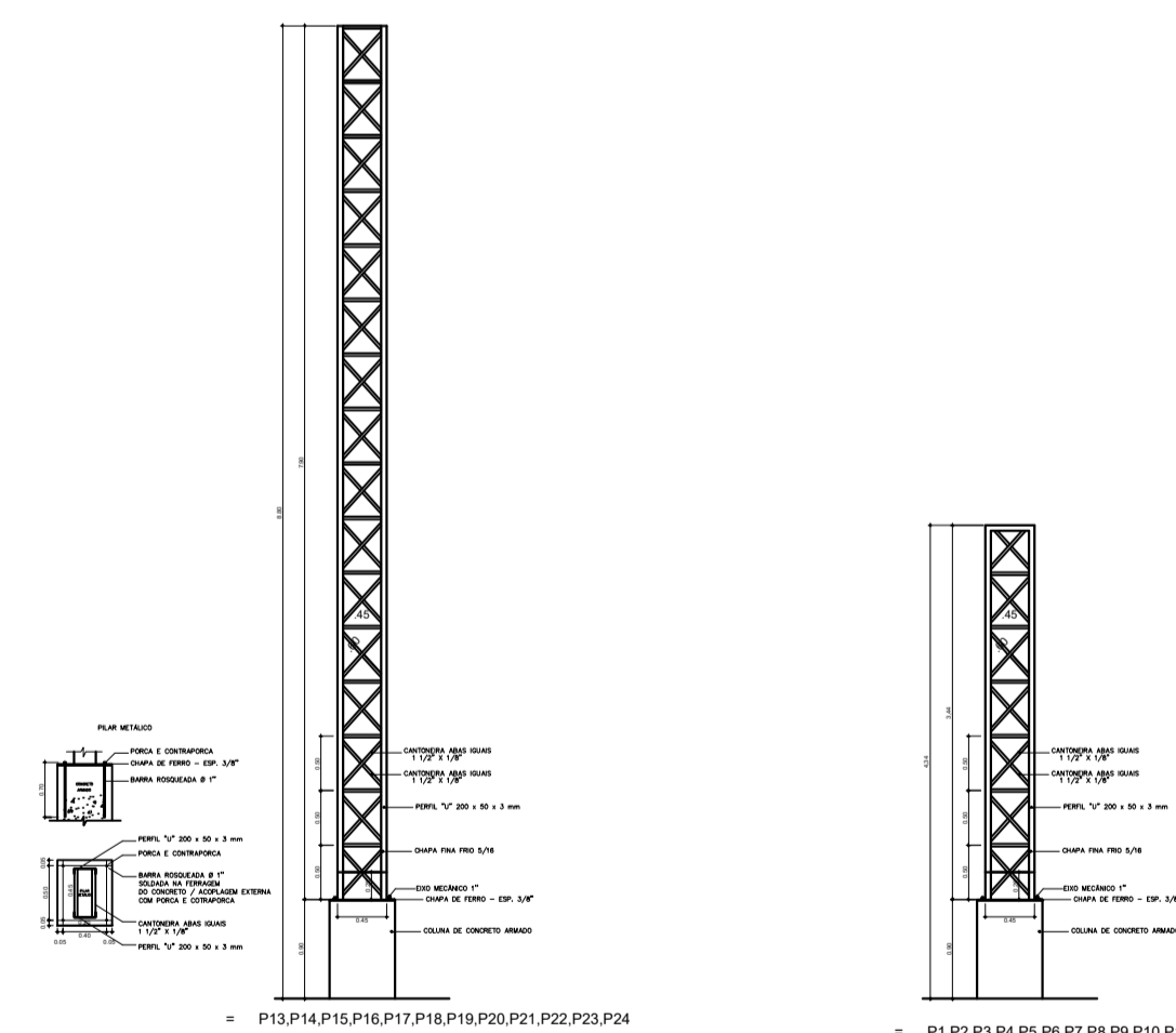
DETALHE DO PILAR METÁLICO 1:75
