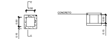
DET. CAIXA RALO ( D.I 0.50 x 0.50 x 0.50 ) ESC. 1/25
