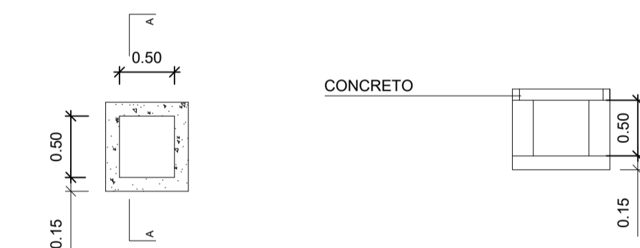
DET. CAIXA RALO ( D.I 0.50 x 0.50 x 0.50 ) ESC. 1/25
