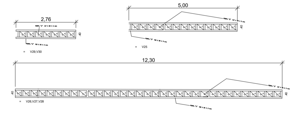
DETALHE TRELIÇA METÁLICA 1:100
