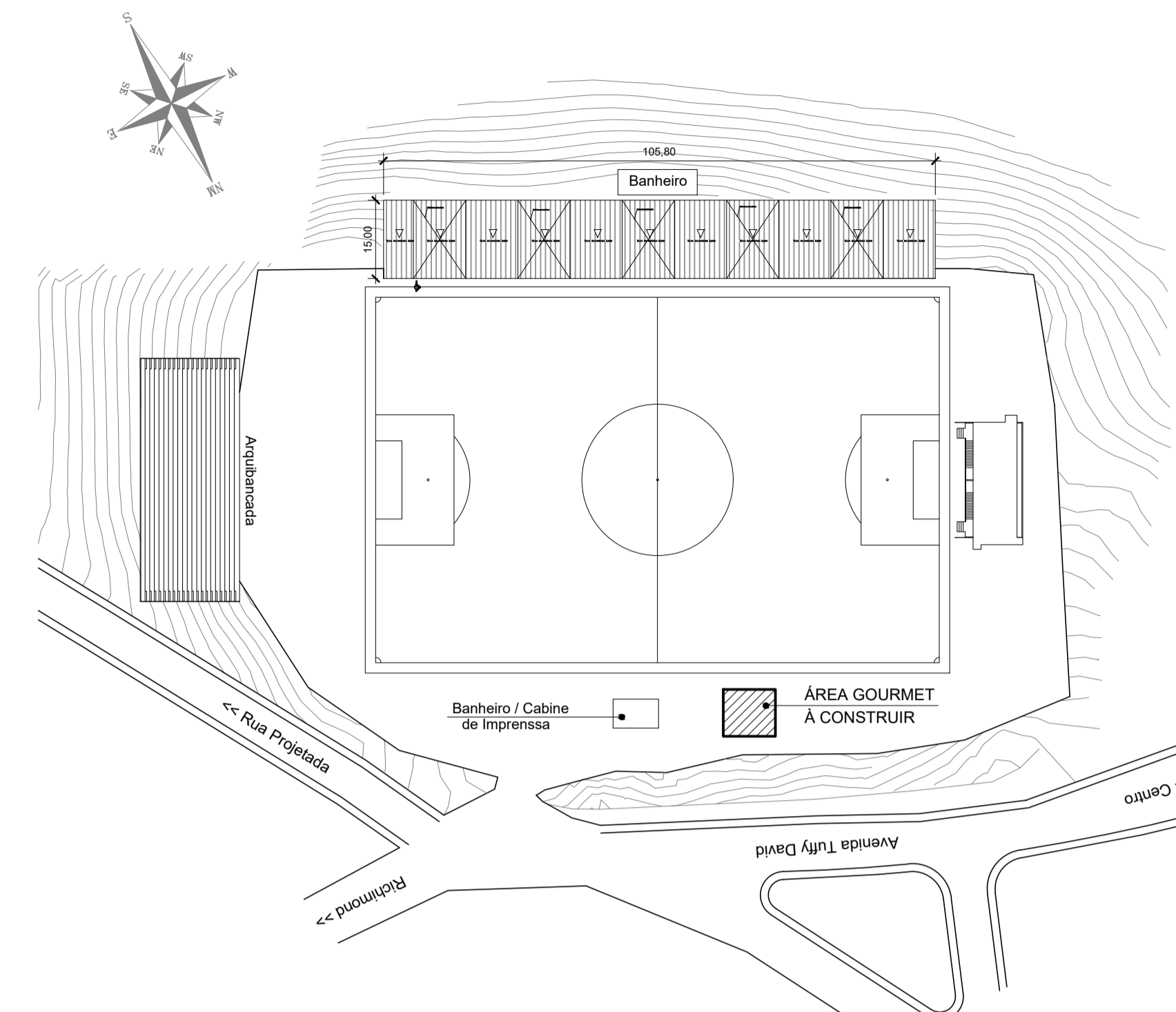
Arquitetura PLANTA DE SITUAÇÃO
