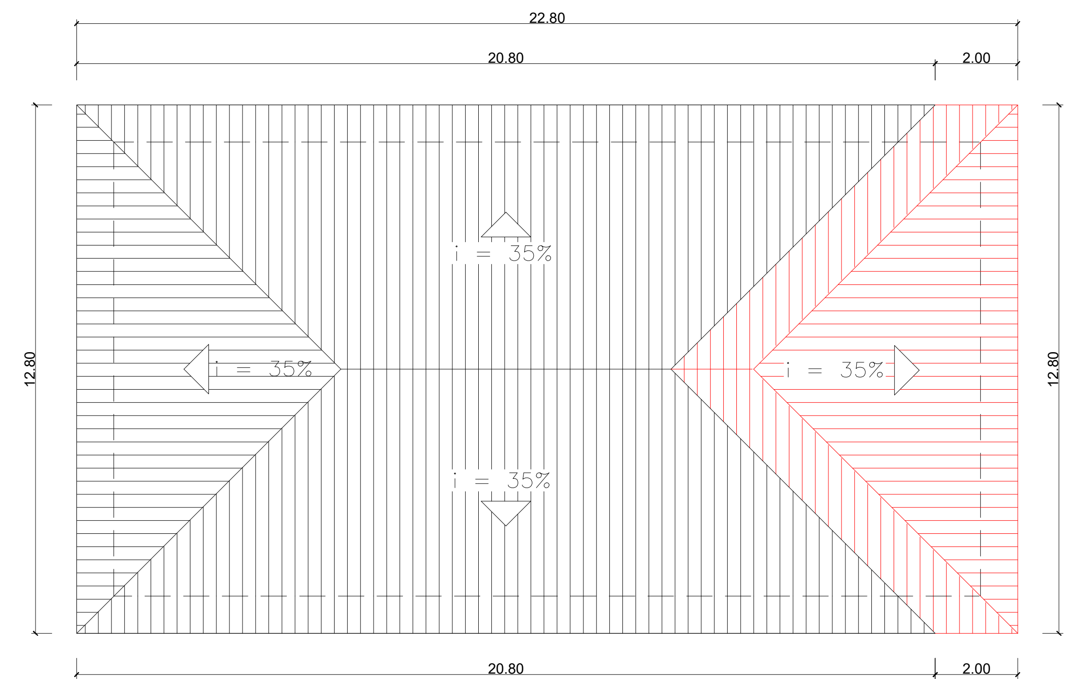
05 PLANTA DE COBERTURA Esc.: 1:125
