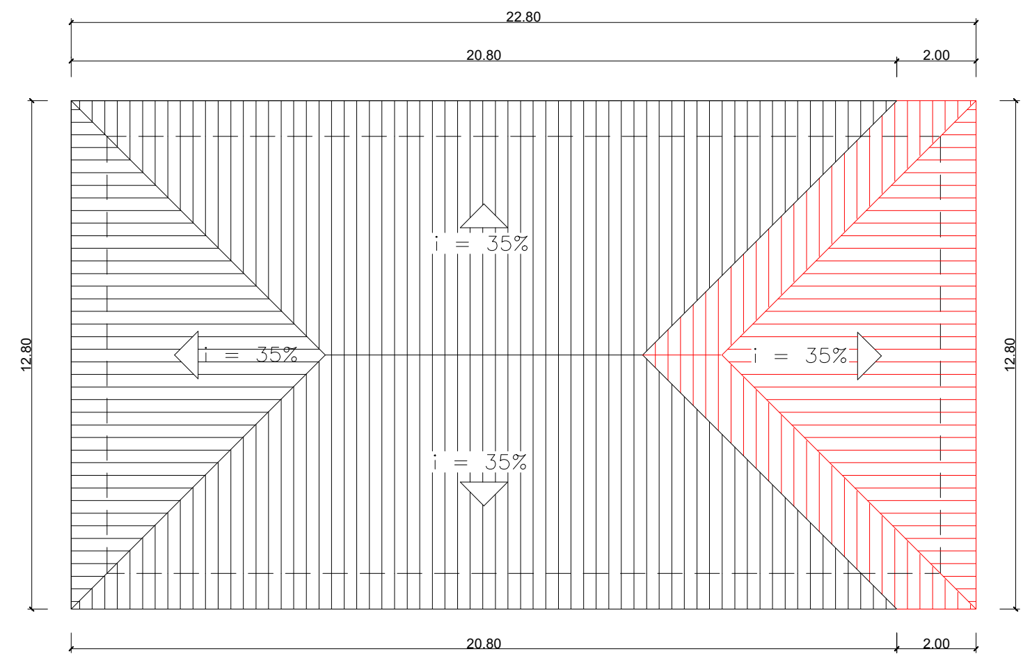
05 PLANTA DE COBERTURA Esc.: 1:125
