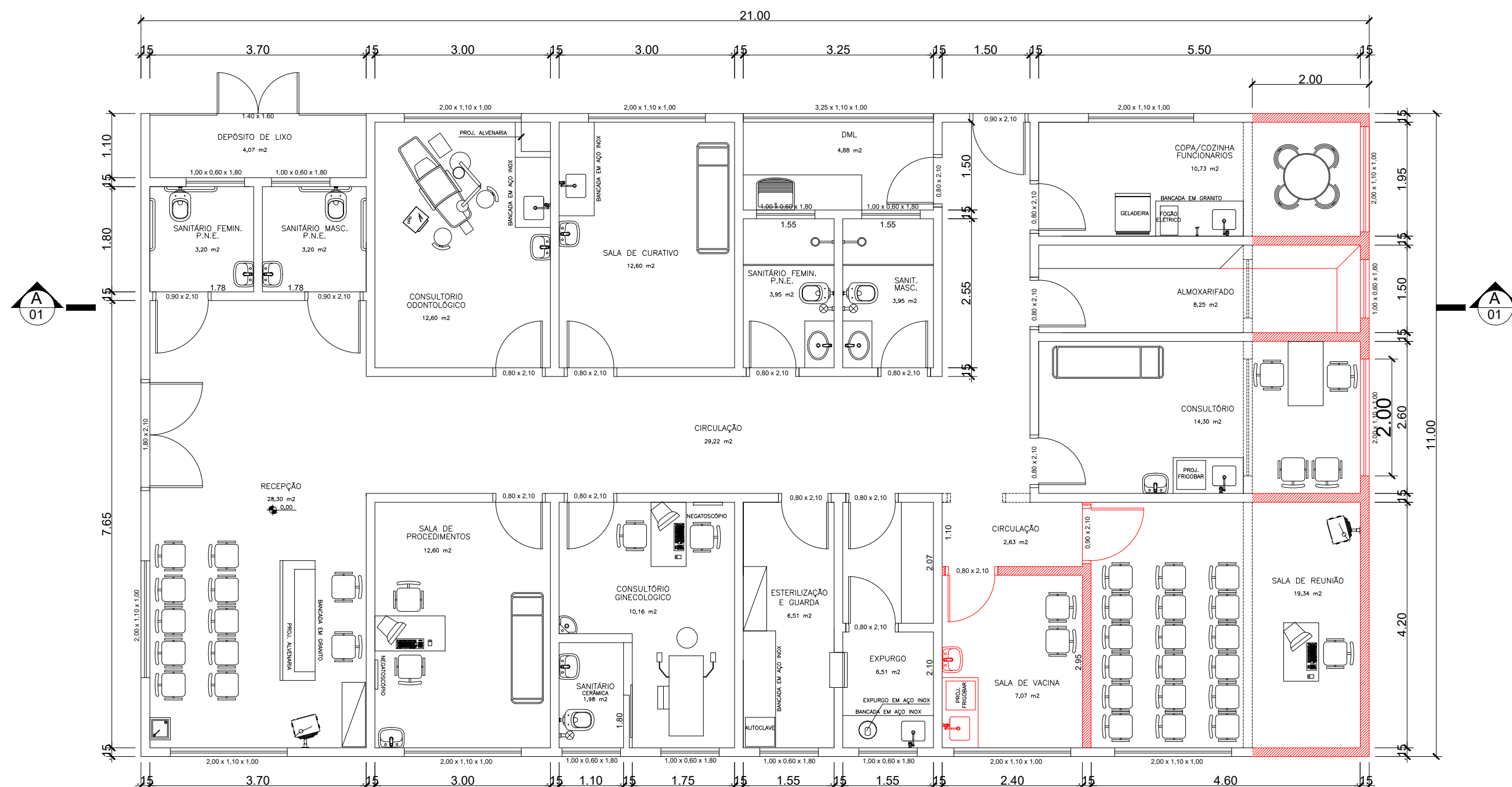
01 PLANTA BAIXA Esc.: 1/75
