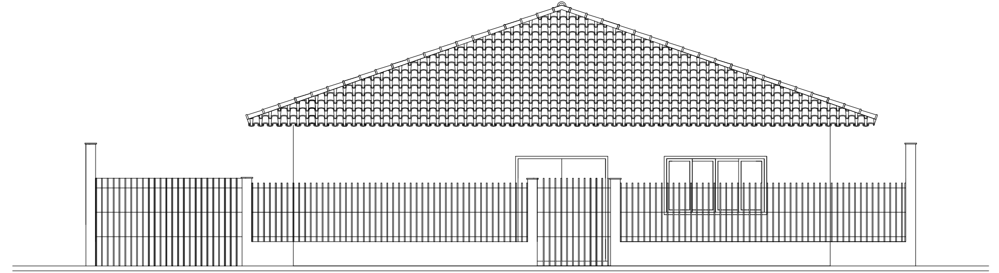
04 FACHADA FRONTAL Esc.: 1/75
