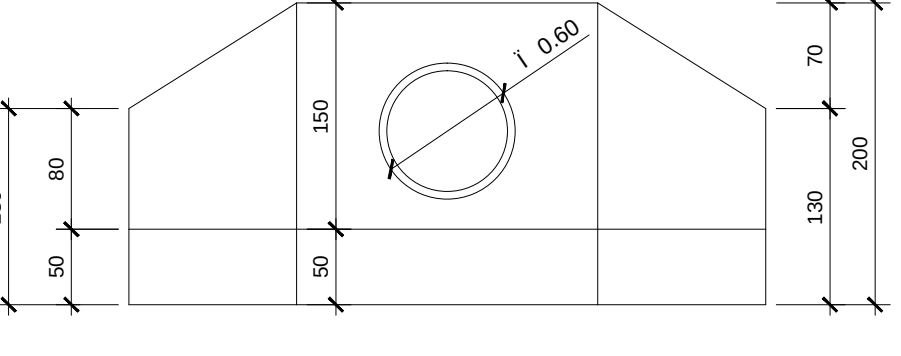
DETALHE - BOCA DE SAÍDA Cotas em metro Escala - 1/50
