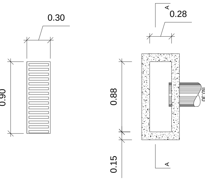
DETALHE - CAIXA RALO Cotas em metro Escala - 1/25
