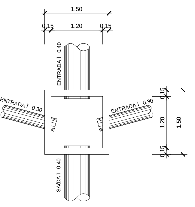
CAIXA DE PASSAGEM - PO&O DE VISITA Cotas em metro Escala - 1/50
