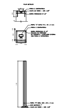
DETALHE DO PILAR METÁLICO 1:50
