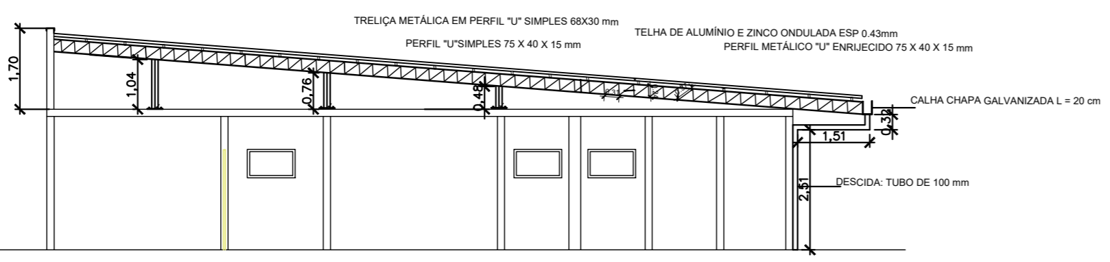
CORTE A-A 1:100
