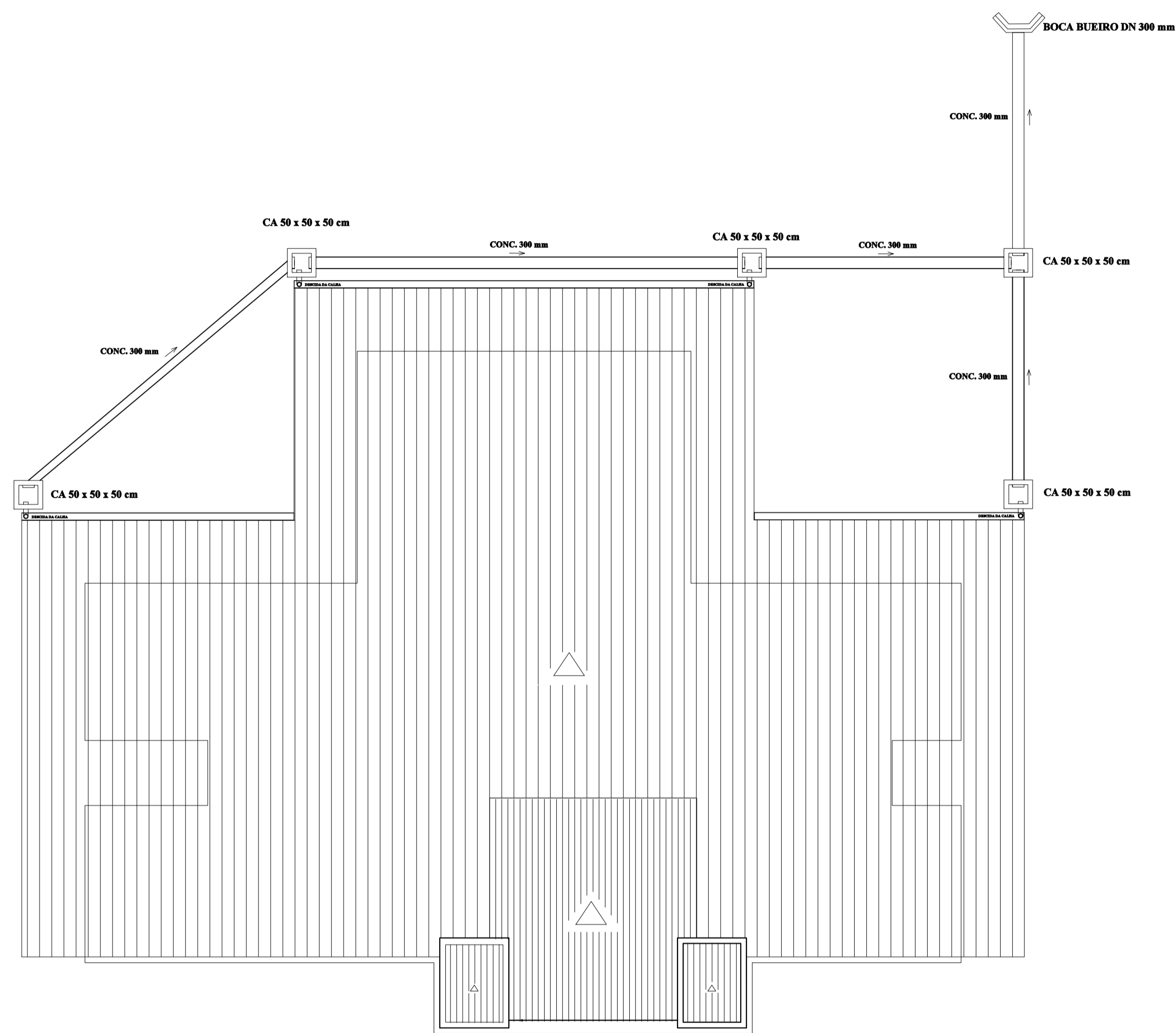
PLANTA BAIXA - DRENAGEM DE ÁGUAS PLUVIAIS Cotas em metro. Escala 1/100
