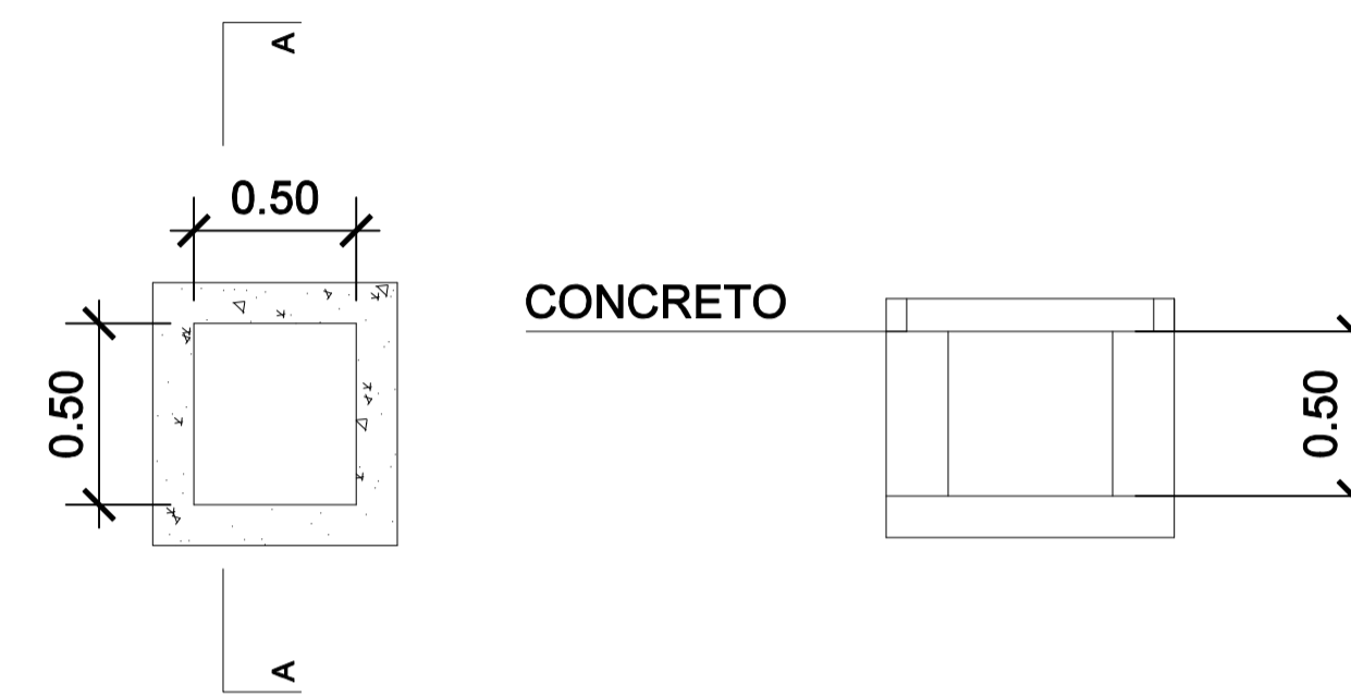
DETALHE - CAIXA DE PASSAGEM 50 X 50 X 50 CM Cotas em metro. Escala 1/25
