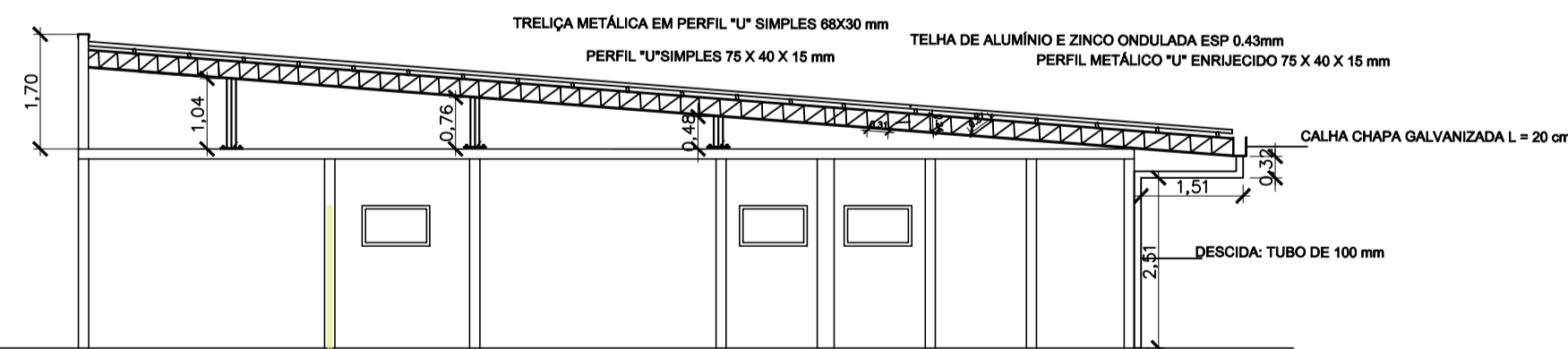
CORTE A-A Cotas em metro. Escala 1/100
