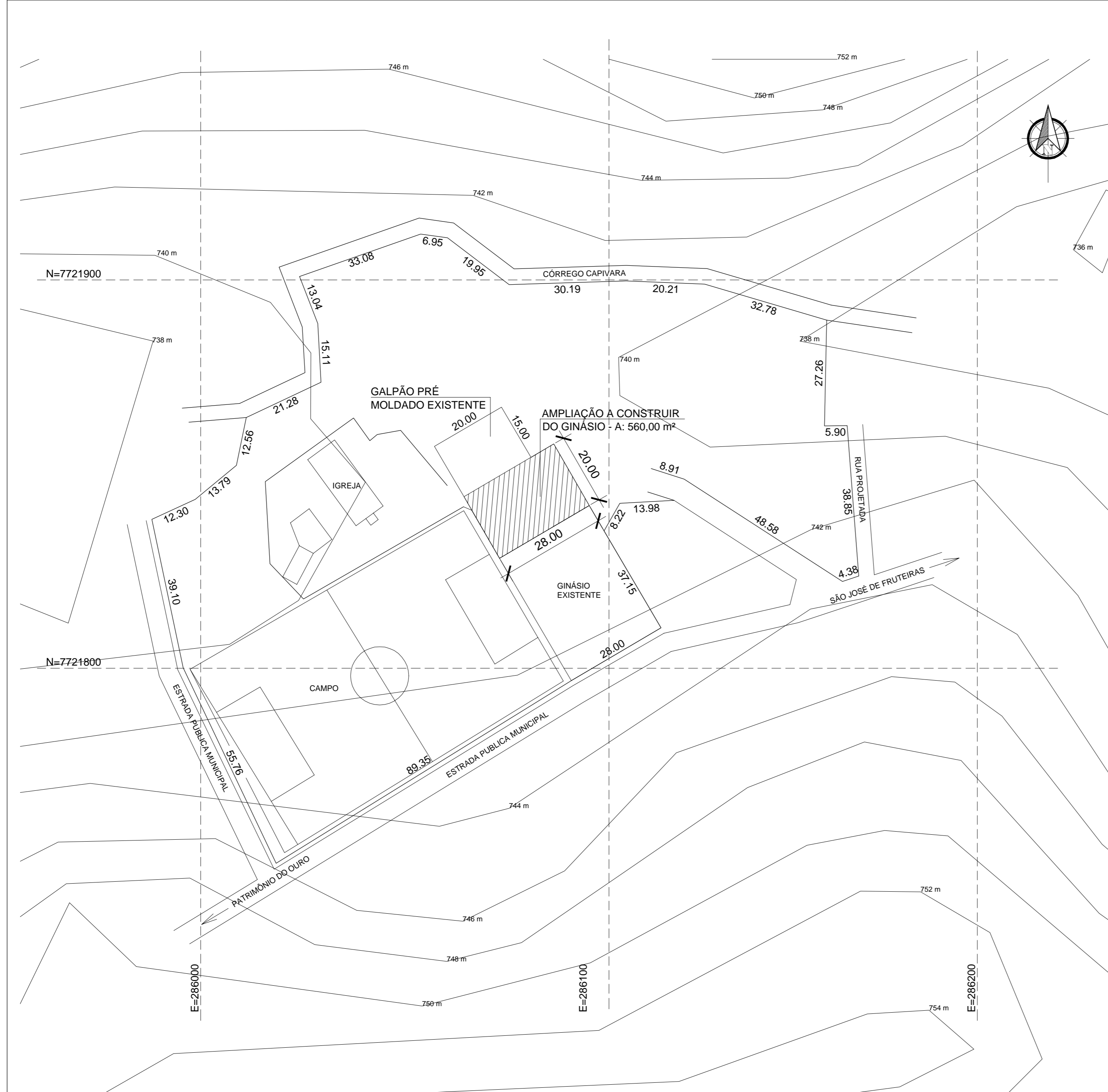
PLANTA DE LOCALIZAÇÃO/SITUAÇÃO Cotas em metro. Escala - 1/750
