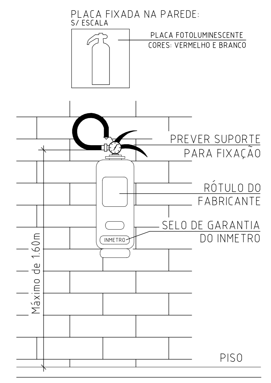
Arquitetura EXTINTOR - SINALIZAÇÃO EM PAREDE Cotas em metros. Escala 1/50
