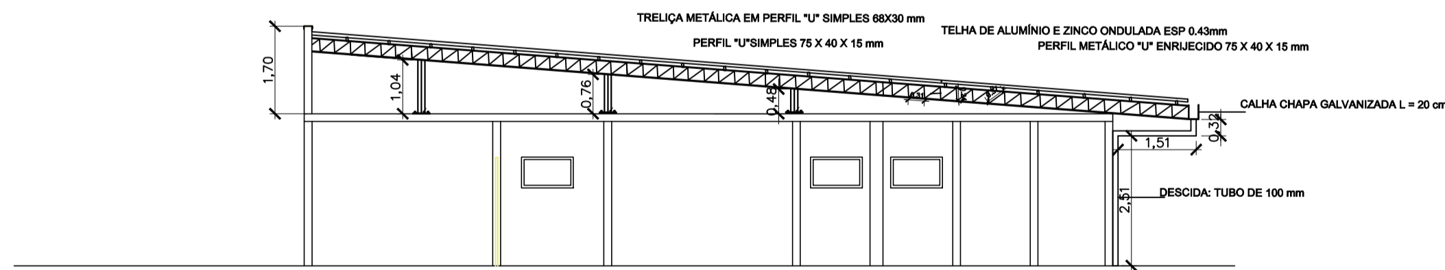
CORTE A-A Cotas em metro. Escala 1/100
