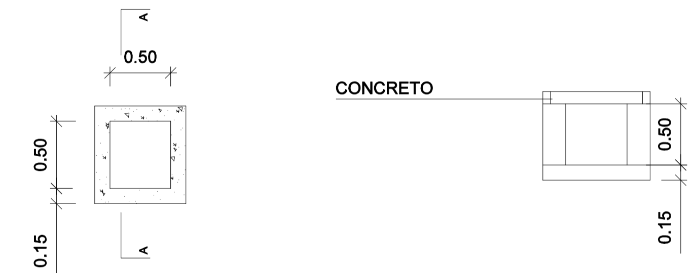
DET. CAIXA RALO ( D.I 0.50 x 0.50 x 0.50 ) ESC. 1/25
