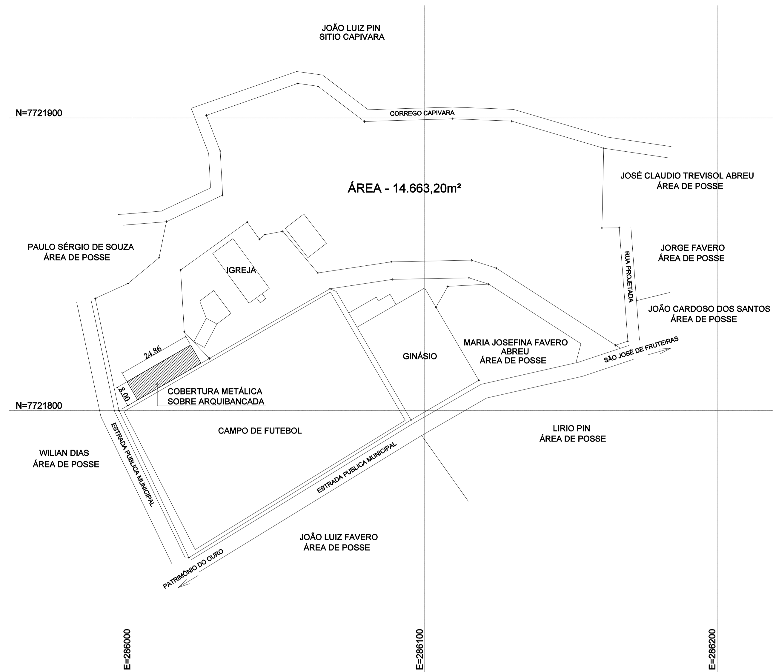
PLANTA DE SITUAÇÃO 1:500
