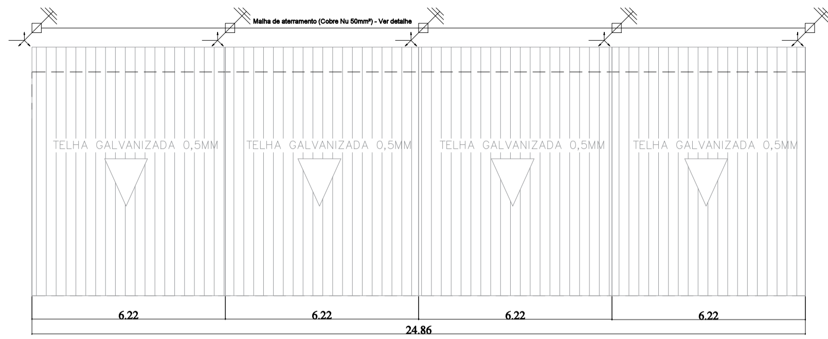
PLANTA BAIXA SPDA 1 : 50
