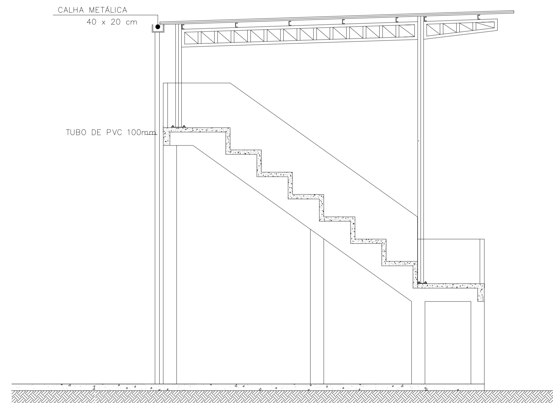
CORTE - A A TUBO DE DRENAGEM 1 : 50
