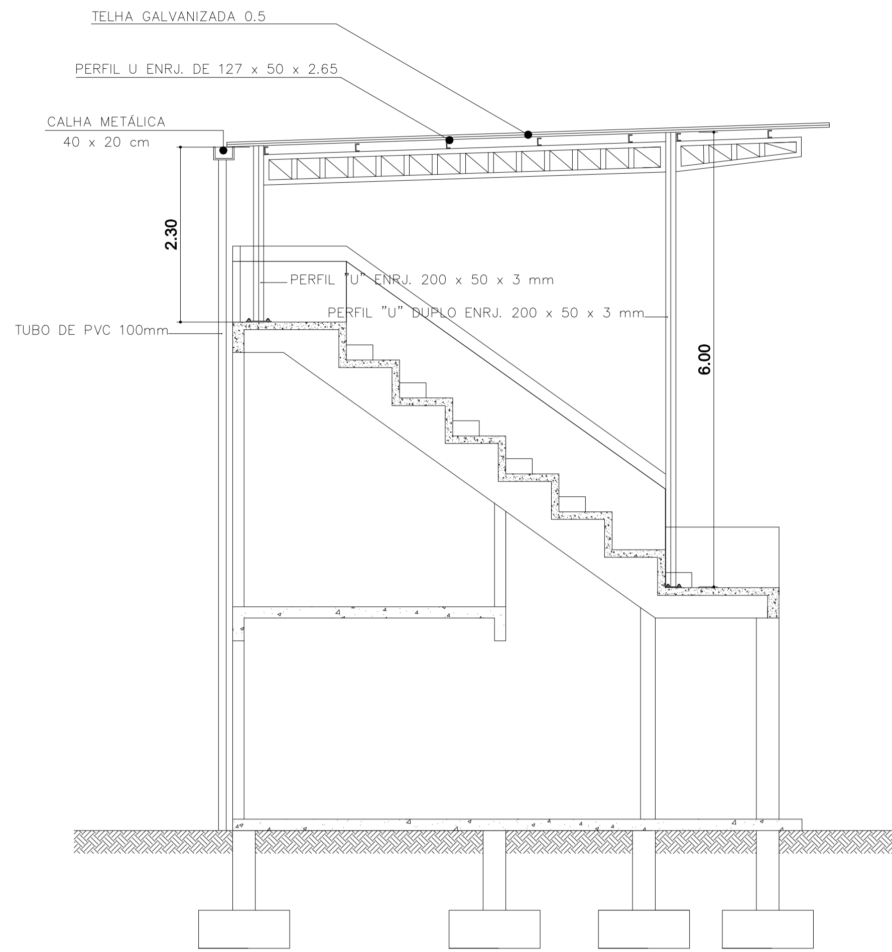
CORTE - A A 1:50
