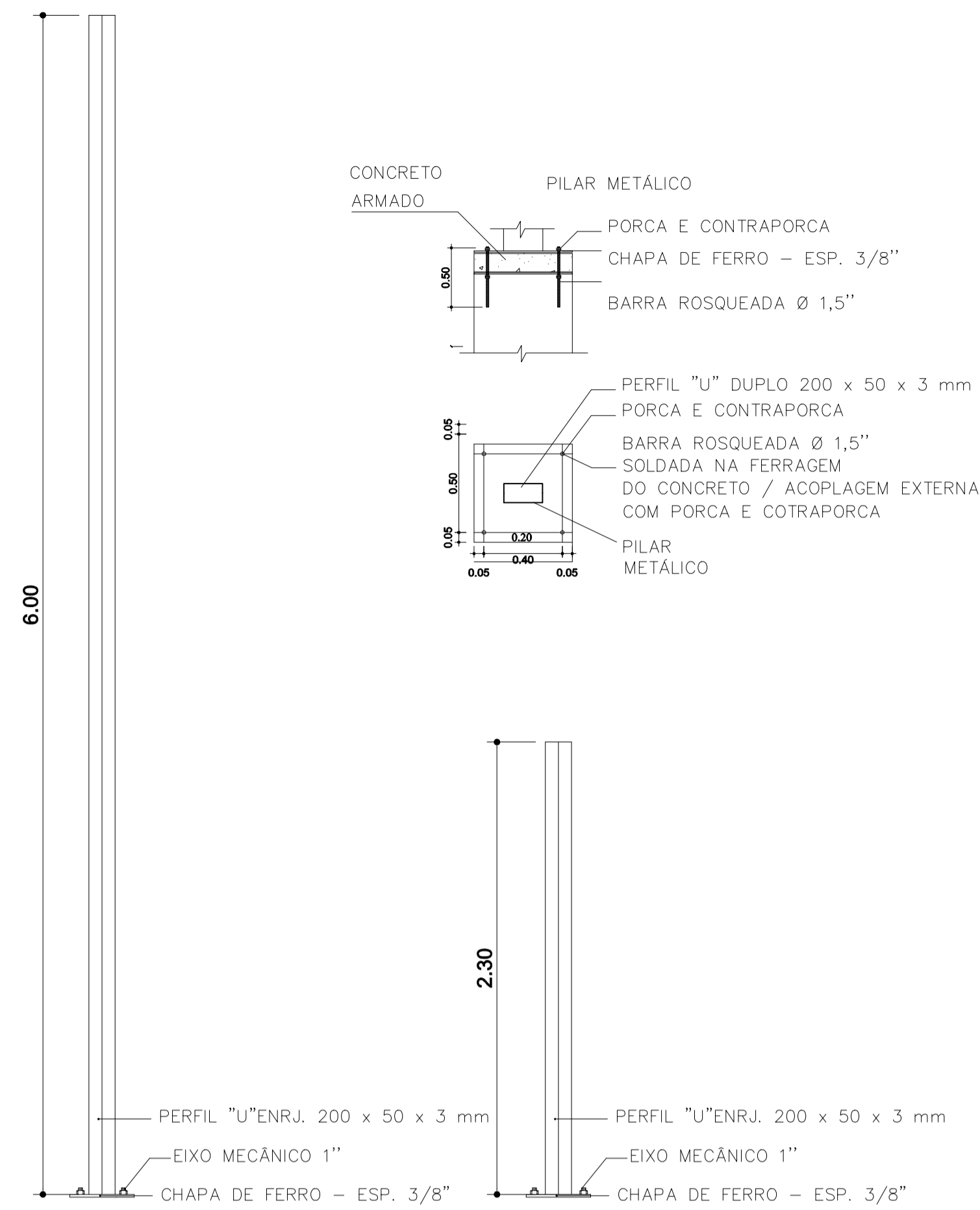
DETALHE DO PILAR METÁLICO 1:25
