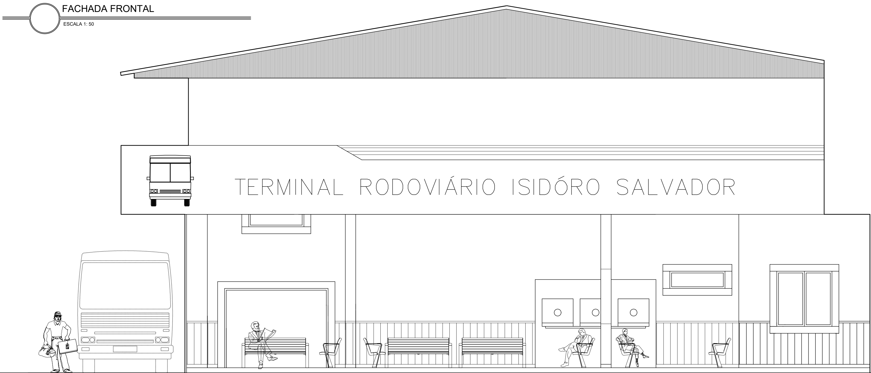
FACHADA FRONTAL - REFORMA ESCALA 1: 50
