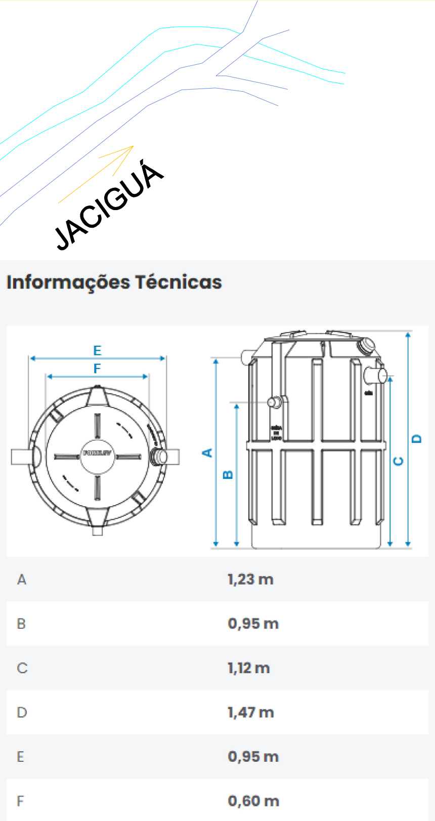
DETALHE DO BIODIGESTOR Cotas em metro. Escala - Sem
