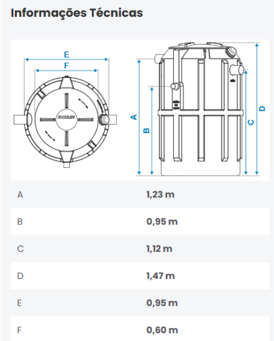
DETALHE DO BIODIGESTOR Cotas em metro. Escala - Sem
